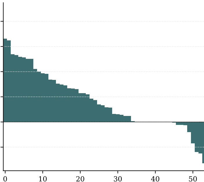
TREC DL20
