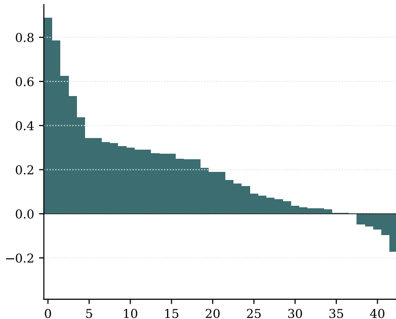
TREC DL19
