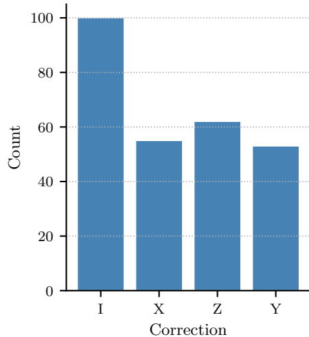
3-qubit errors (270)
