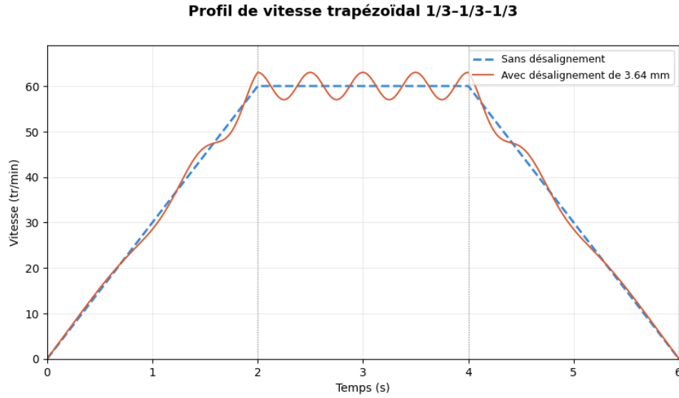
Figure 6.1 – Profil de vitesse trapézoïdal 1/3-1/3-1/3 avec saccade périodique due au désalignement de l'accouplement fourche-T.
