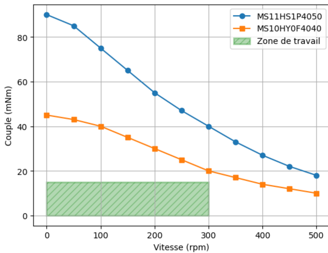
Figure 5.1 – Courbes couple-vitesse des moteurs NEMA
