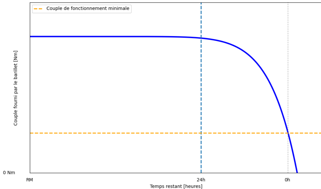
Figure 2.1 – Évolution du couple fourni par le barillet en fonction du temps
