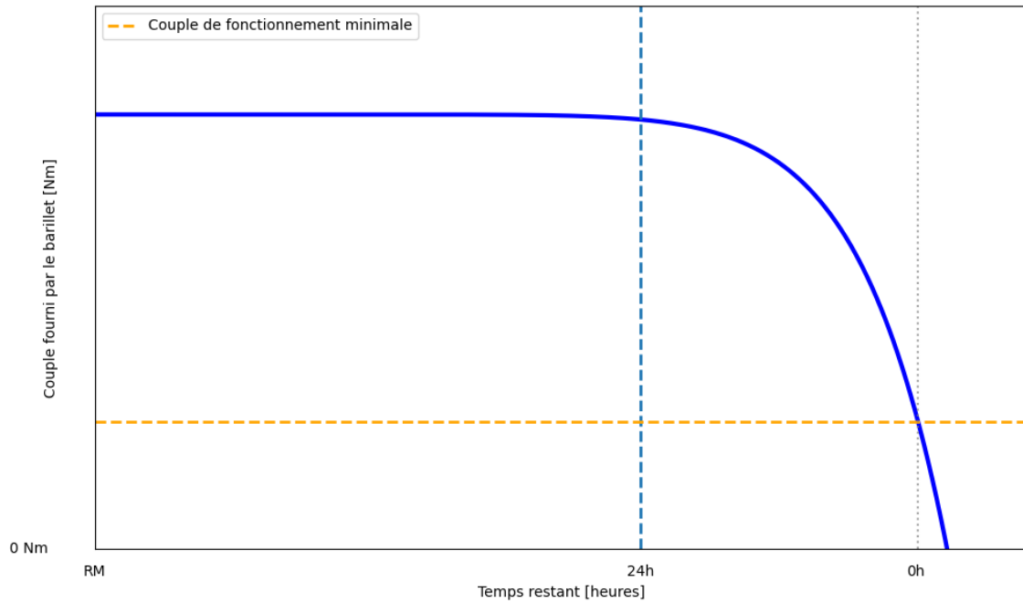
Figure 2.4 – Évolution du couple fourni par le barillet en fonction du temps
