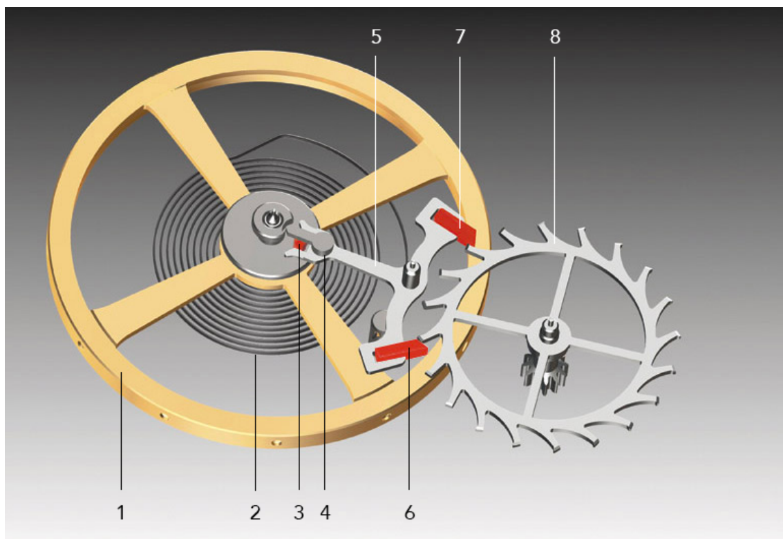
Figure 2.3 – Illustration d'un échappement à ancre suisse trouvé sur le site de Worldtempus [5]
