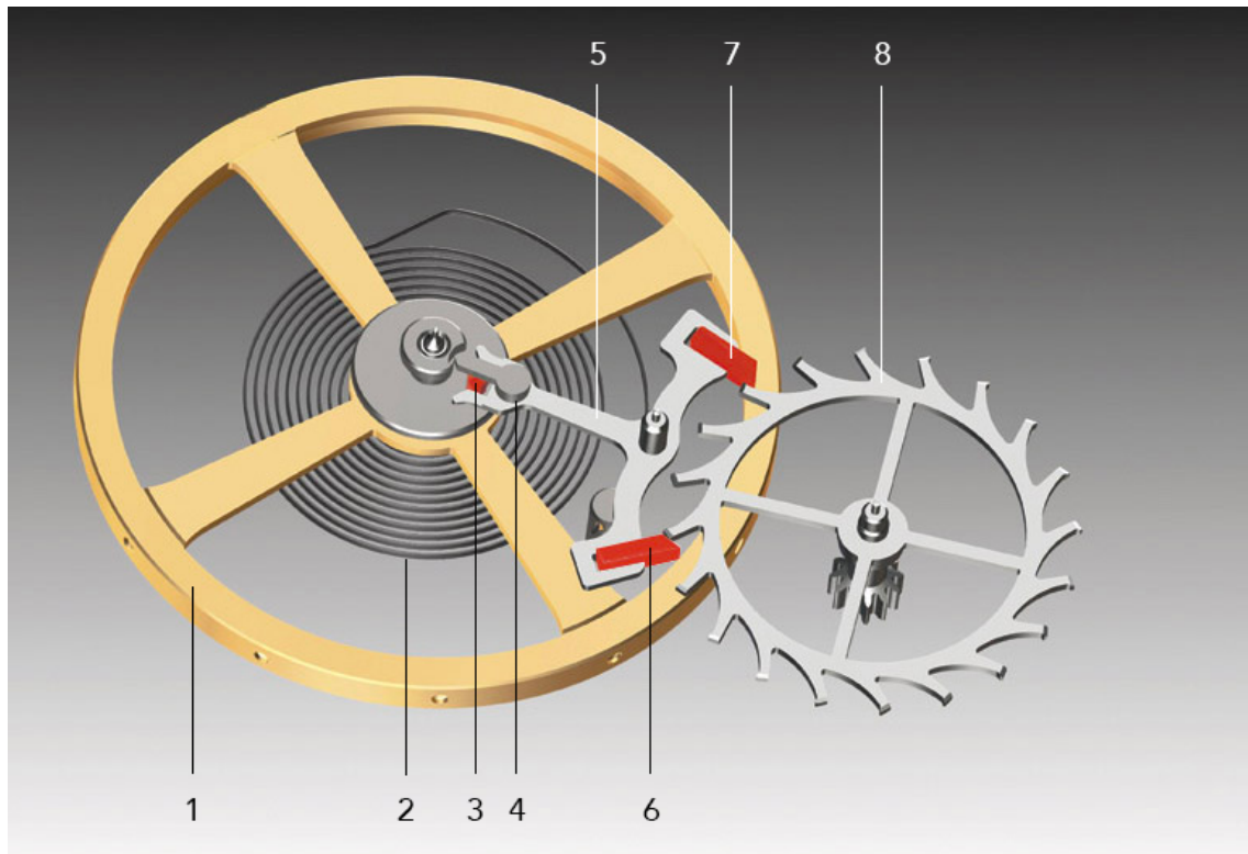
Figure 2.3 – Illustration d'un échappement à ancre suisse trouvé sur le site de Worldtempus [Worldtempus]
