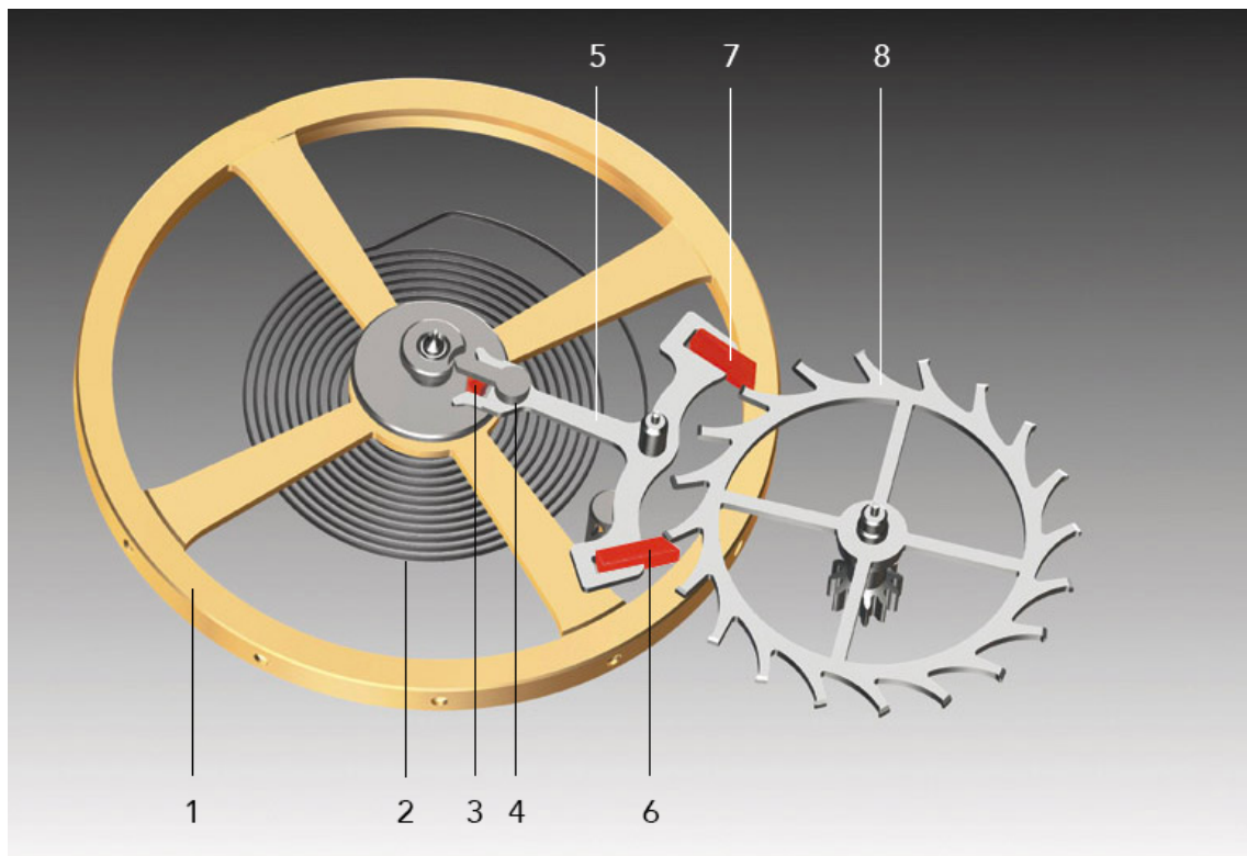
Figure 2.3 – Illustration d'un échappement à ancre suisse trouvé sur le site de Worldtempus [5]
