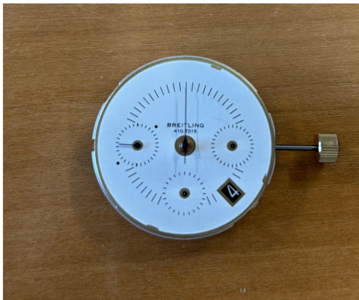
Figure 5.2 – Mouvement dans la configuration de mesure COSC
