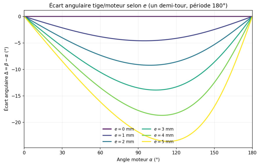
Figure 6.17 – Écart angulaire \Delta = \beta - \alpha sur un demi-tour, pour différentes valeurs du désalignement e (0 à 5 mm). Ce motif se répète à l'identique tous les 180^\circ (et non tous les 360^\circ ), conséquence directe de la symétrie de la fourche en T .
