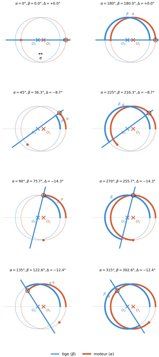
Figure 6.15 – Position de la tige (bleu, angle \beta ) en fonction de la position du moteur (orange, angle \alpha ), tous les 45^\circ sur un tour complet, en deux colonnes de quatre. Les axes O_1 (moteur) et O_2 (tige) et leur désalignement e sont indiqués sur le premier panneau; le bras moteur actif est entouré. R = 12,5 \text{ mm} , e = \Delta h = 3,18 \text{ mm} .
