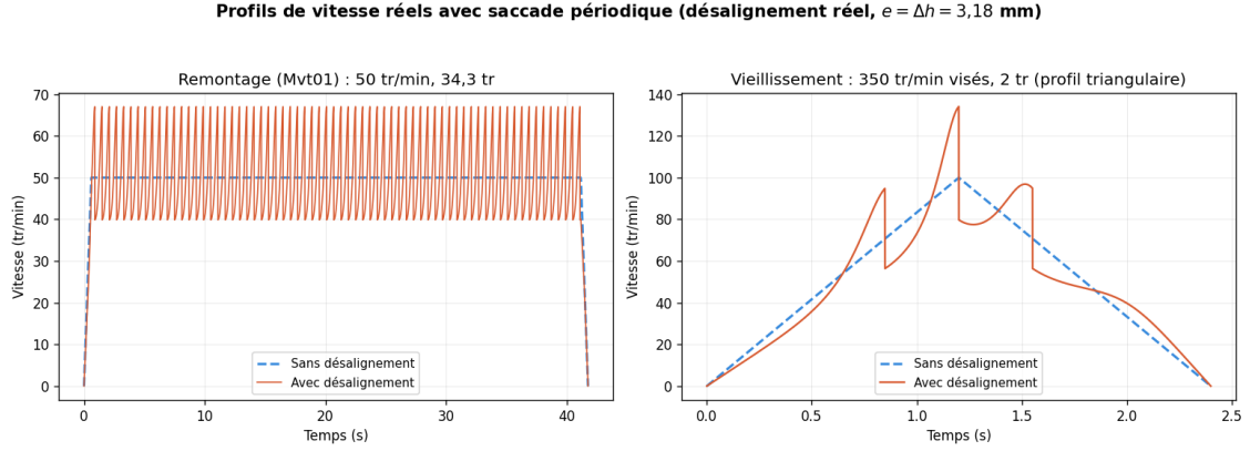
Figure 6.18 – Profils de vitesse réels avec saccade périodique due au désalignement réel de l'accouplement, e = \Delta h = 3,18 mm : remontage du Mvt01 (gauche) et vieillissement accéléré (droite, profil triangulaire). Le motif se répète tous les 180^\circ de rotation moteur.
