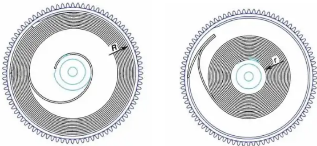
(a) Ressort désarmé
