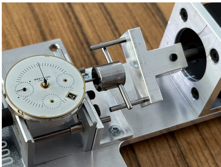
Figure 5.4 – Accouplement fourche-T assemblé entre le moteur et la tige du mouvement
