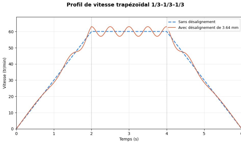
Figure 6.15 – Profil de vitesse trapézoïdal 1/3-1/3-1/3 avec saccade périodique due au désalignement de l'accouplement fourche-T.
