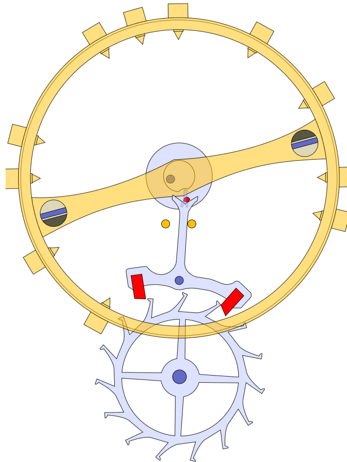
Figure 2.5 – Échappement à ancre suisse [Worldtempus]
