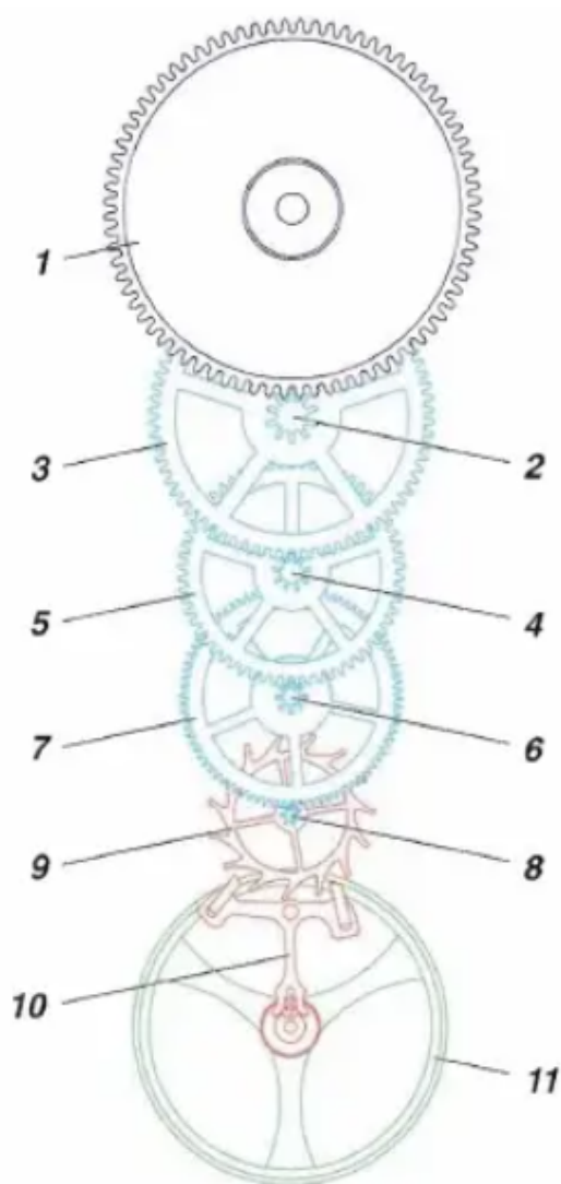
Figure 2.1 – Transmission de l'énergie dans un mouvement de montre [theorie_horlogerie/
