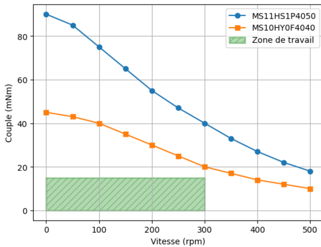
Figure 5.1 – Courbes couple-vitesse des moteurs NEMA
