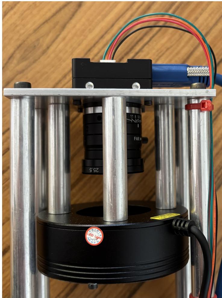
Figure 5.6 – Caméra et ring light positionnées au-dessus du mouvement en test
