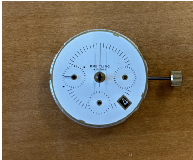
Figure 5.2 – Mouvement dans la configuration de mesure COSC
