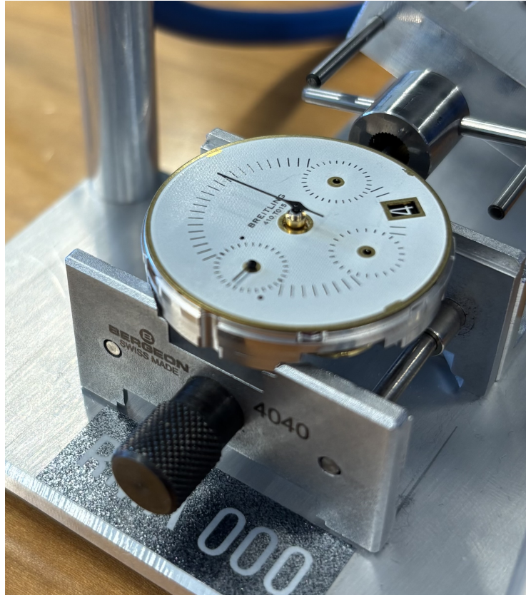
Figure 5.3 – Porte-mouvement avec un calibre en position de test
