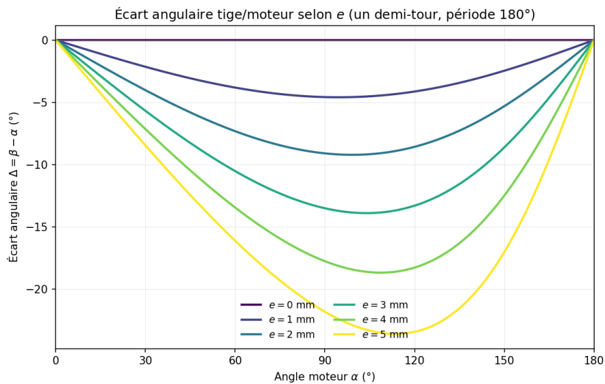
Figure 6.17 – Écart angulaire \Delta\theta = \beta - \alpha sur un demi-tour, pour différentes valeurs du désalignement e (0 à 5 mm). Ce motif se répète à l'identique tous les 180^\circ (et non tous les 360^\circ ), conséquence directe de la symétrie de la fourche en U.
