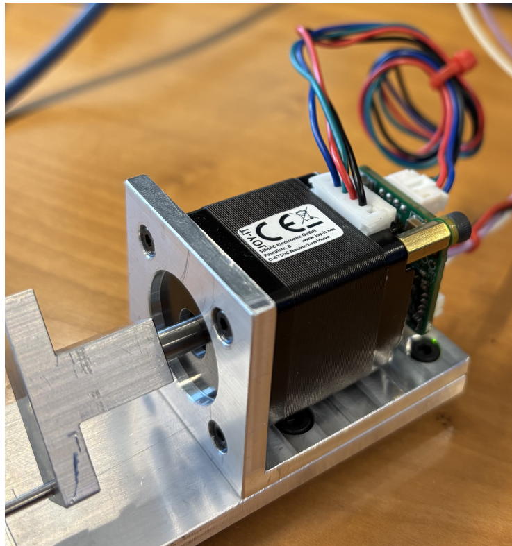
Figure 5.4 – Moteur pas à pas NEMA 11 monté sur la structure
