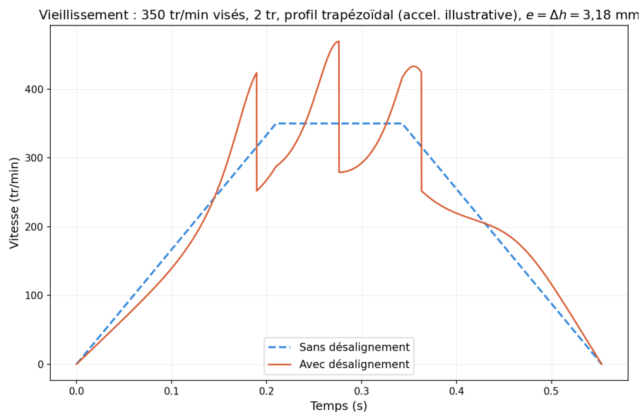
Figure 6.19 – Profil de vitesse illustratif en mode vieillissement accéléré (accélération de 100 000 tr/min 2 , non représentative du système réel), avec saccade périodique due au désalignement e = \Delta h = 3,18 mm.
