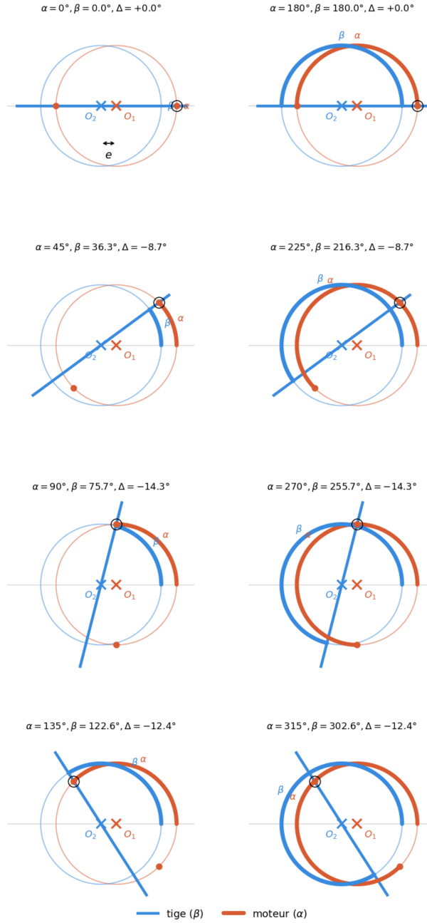
Figure 6.15 – Position de la tige (bleu, angle \beta ) en fonction de la position du moteur (orange, angle \alpha ), tous les 45^\circ sur un tour complet, en deux colonnes de quatre panneaux. Les axes O_1 (moteur) et O_2 (tige) et leur désalignement e sont indiqués sur le premier panneau; la goupille active de la fourche en U est entourée. R = 12,5 \text{ mm} , e = \Delta h = 3,18 \text{ mm} .
