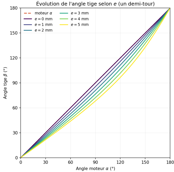
Figure 6.16 – Évolution de l'angle tige \beta sur un demi-tour, pour différentes valeurs du désalignement e (0 à 5 mm). Le désalignement réel ( \Delta h = 3,18 mm) se situe entre les courbes e = 3 mm et e = 4 mm. Le comportement se répète à l'identique sur chaque demi-tour suivant.
