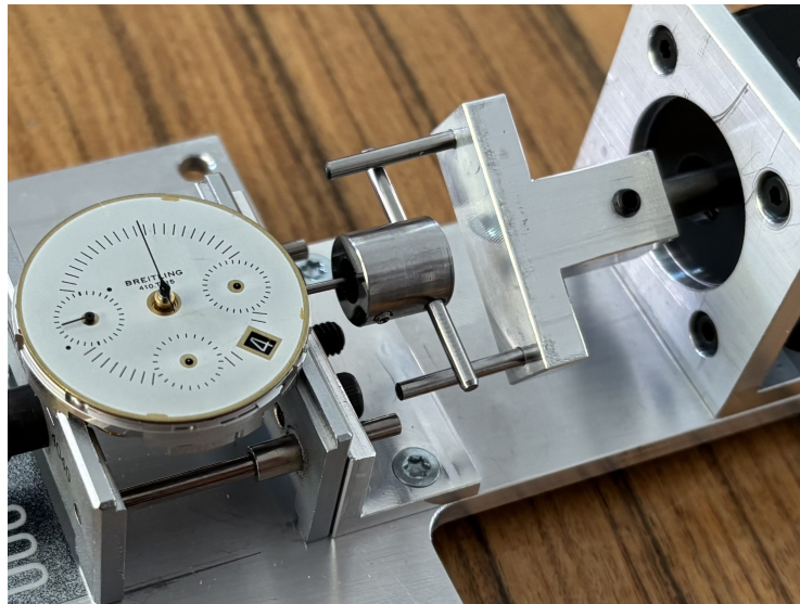
Figure 5.5 – Accouplement fourche en T – fourche en U assemblé entre le moteur et la tige du mouvement
