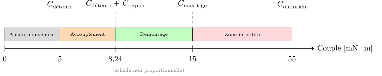
Figure 6.5 – Plages de couple et régimes de fonctionnement du moteur
