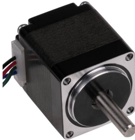
Figure 6.3 – Moteur pas à pas NEMA11-01 de Joy-IT [16]
