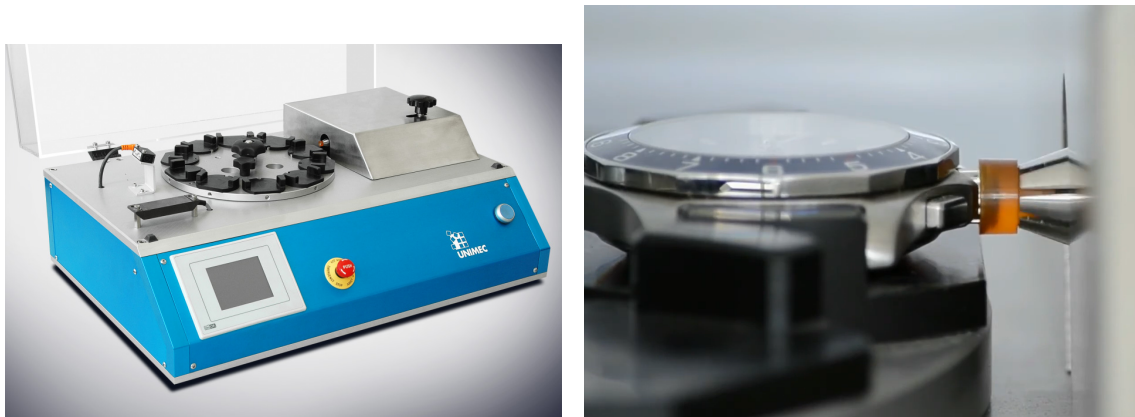
Figure 4.3 – Machine de remontage de montres d'UNIMEC SA [12]
