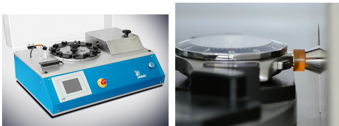
Figure 4.3 – Machine de remontage de montres d'UNIMEC SA [9]
