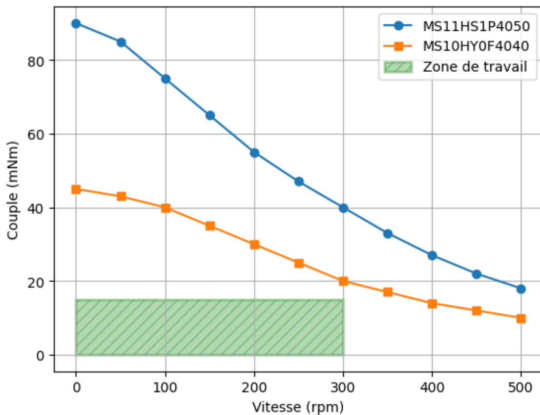
Figure 5.3 – Courbes couple-vitesse des moteurs NEMA
