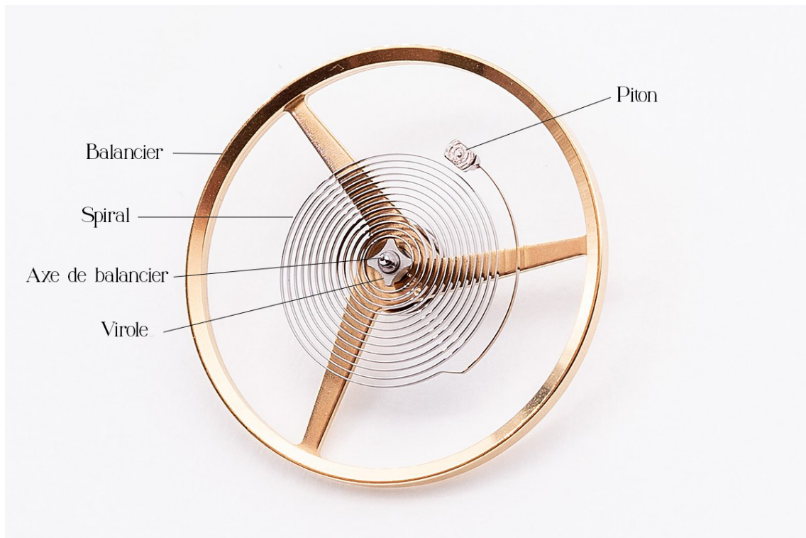
Figure 2.2 – Illustration d'un balancier et du spiral trouvé sur le site de Elégance et précision [4]
