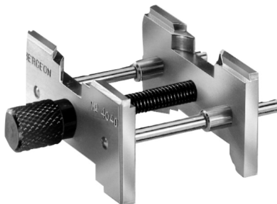
Figure 5.1 – Illustration du porte mouvement N° 4040 issue de la datasheet disponible en annexe [10]
