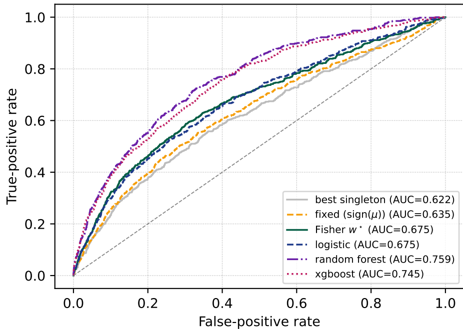
ROC
