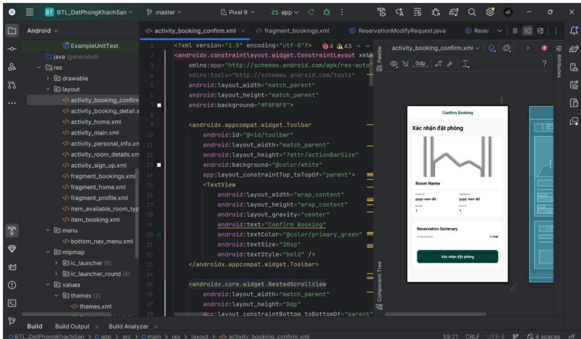
Hình 4.8. Triển khai trang Xác nhận đặt phòng
