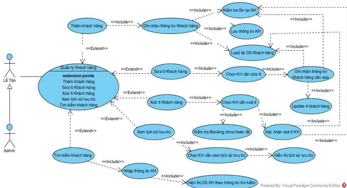
Hình 3.7. Usecase quản lý khách hàng
