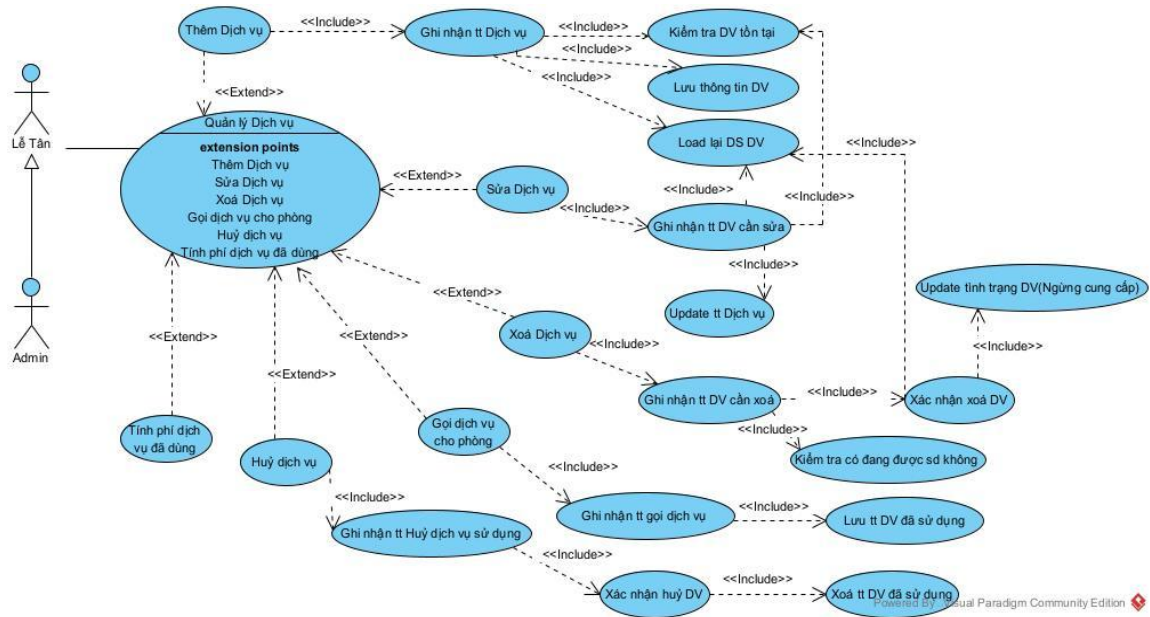
Hình 3.5. Usecase quản lý dịch vụ
