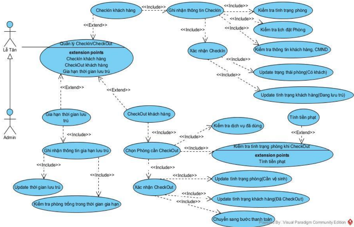
Hình 3.3. Usecase nhận/trả phòng
