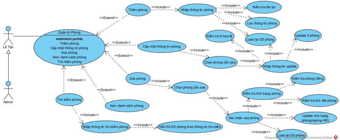
Hình 3.8. Usecase quản lý phòng
