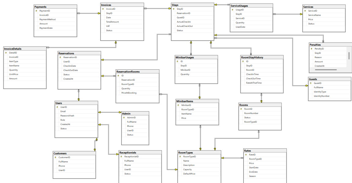
Hình 3.14. Mô hình dữ liệu quan hệ
