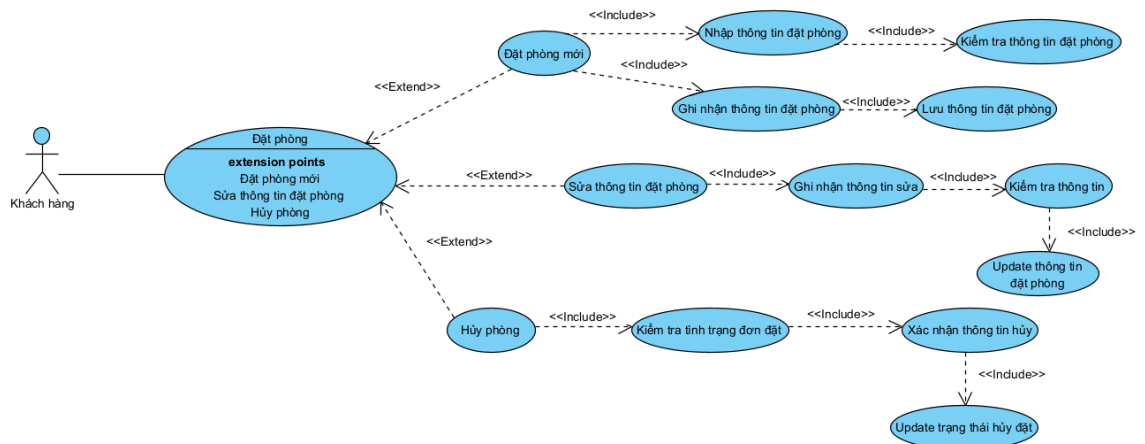
Hình 3.12. Usecase khách hàng đặt phòng
