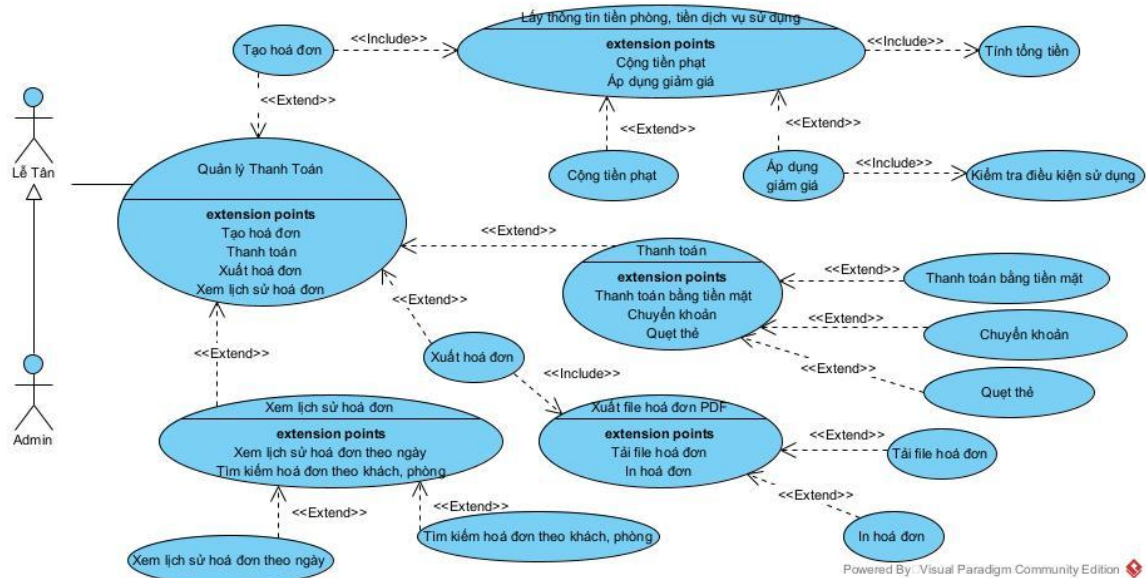
Hình 3.6. Usecase quản lý hóa đơn
