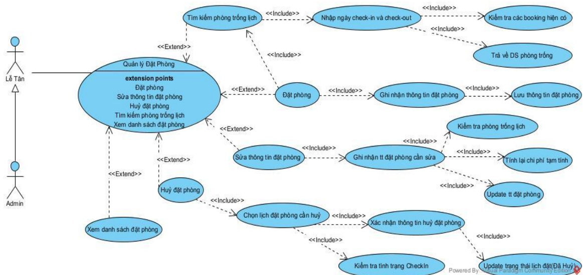
Hình 3.4. Usecase quản lý đặt phòng
