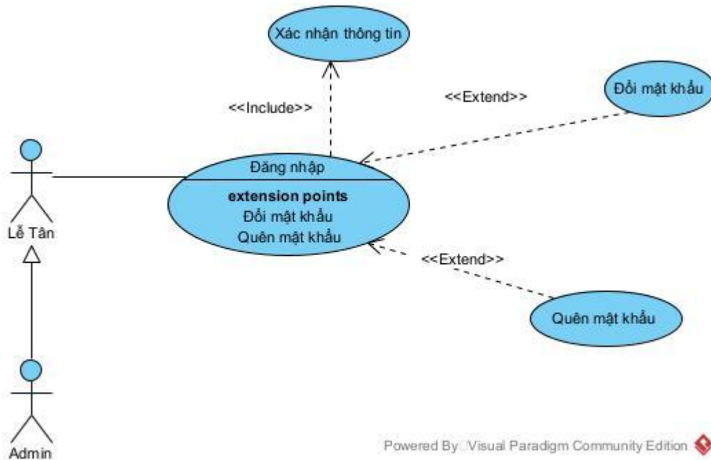
Hình 3.2. Usecase đăng nhập
