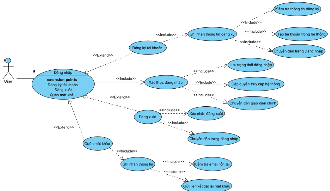
Hình 3.11. Usecase đăng nhập và đăng ký tài khoản
