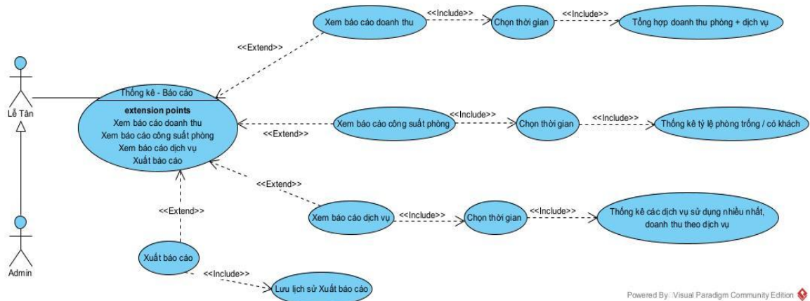
Hình 3.10. Usecase báo cáo thống kê
