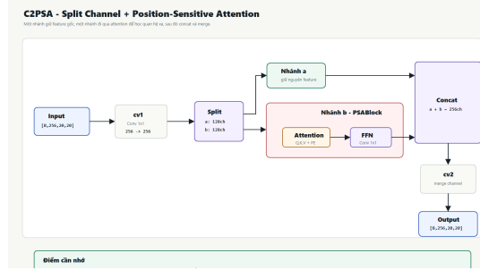
Hình 4.10: Sơ đồ C2PSA: CSP splitting + PSABlock.
