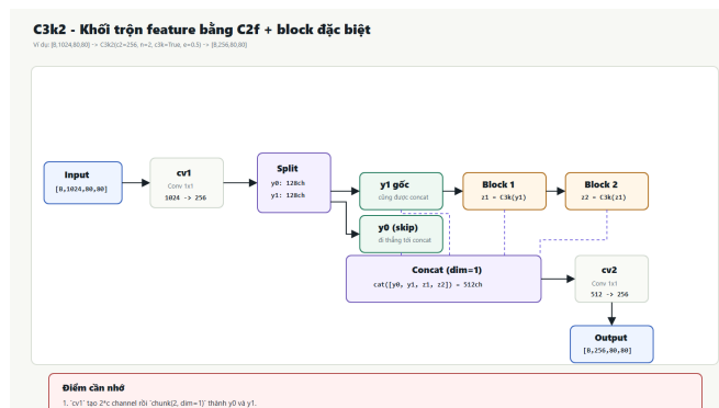
Hình 4.4: Sơ đồ khối C3k2 — forward theo C2f, block bên trong tùy cấu hình.
