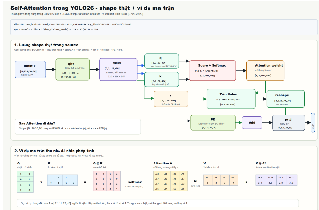
Hình 4.8: Chi tiết luồng xử lý và sự biến đổi kích thước tensor trong module Attention.
