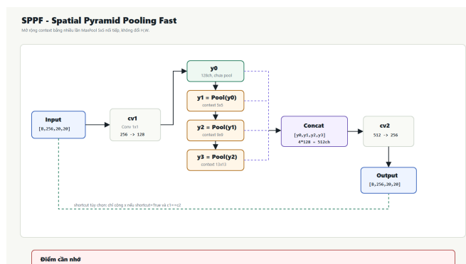
Hình 4.5: Sơ đồ khối SPPF — MaxPool liên tiếp tạo multi-scale receptive field.
