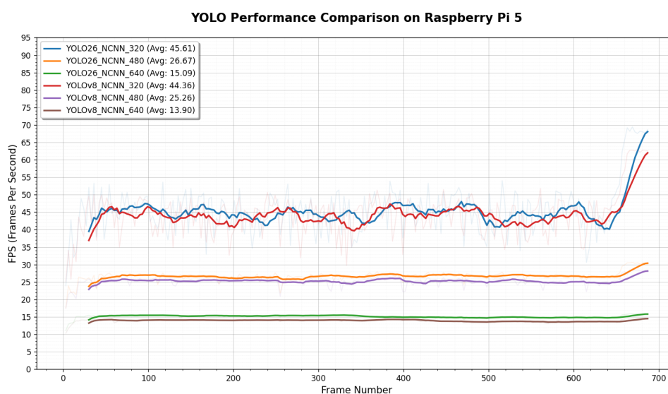
Hình 6.1: So sánh FPS giữa YOLO26 NCNN và YOLOv8 NCNN trên Raspberry Pi 5 ở các độ phân giải đầu vào 320, 480, 640.
