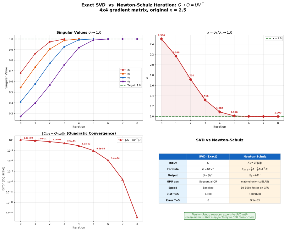
Hình 5.5: Tốc độ hội tụ trực giao hóa của thuật toán lặp Newton-Schulz so với SVD.
