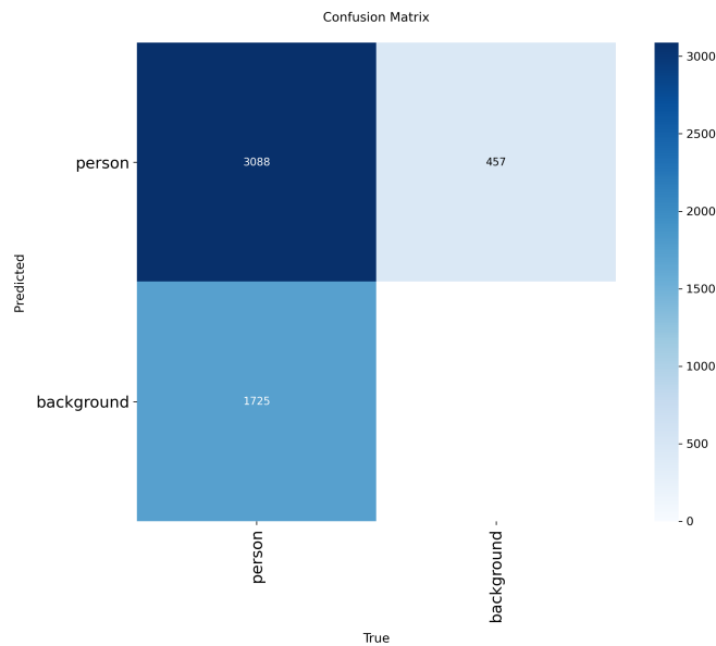
Hình 5.2: Ma trận nhầm lẫn (Confusion Matrix) của YOLO26 gốc trên tập validation.
