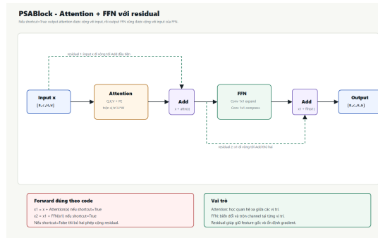
Hình 4.9: Sơ đồ PSABlock: Attention + FFN với các kết nối residual.
