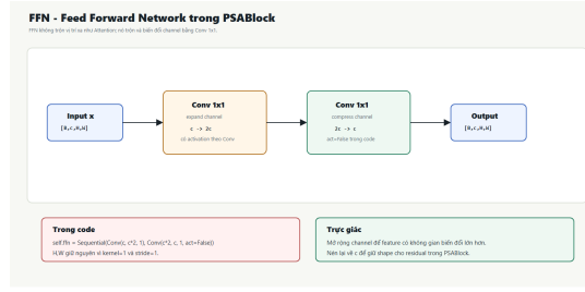
Hình 4.10: Sơ đồ khối FFN (Feed-Forward Network) trong PSABlock.
