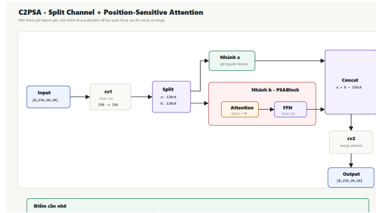
Hình 4.11: Sơ đồ C2PSA: CSP splitting + PSABlock.
