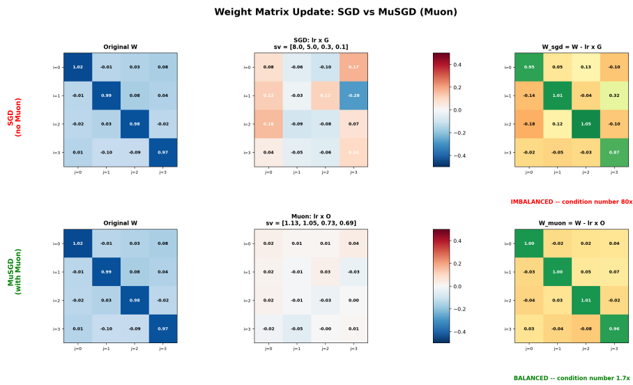
Hình 5.4: So sánh bản chất cập nhật trọng số giữa bộ tối ưu SGD thông thường và Muon (trực giao hóa).
