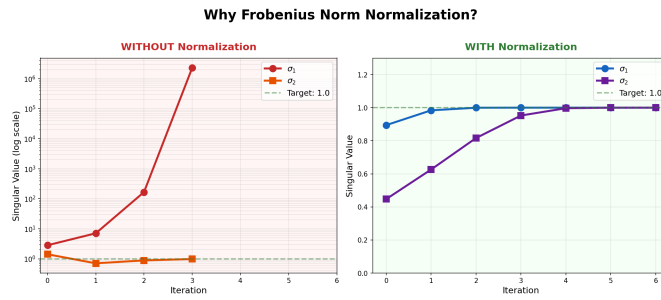
Hình 5.7: Phân tích lý do sử dụng chuẩn Frobenius trong việc khởi tạo thuật toán lặp Newton-Schulz.
