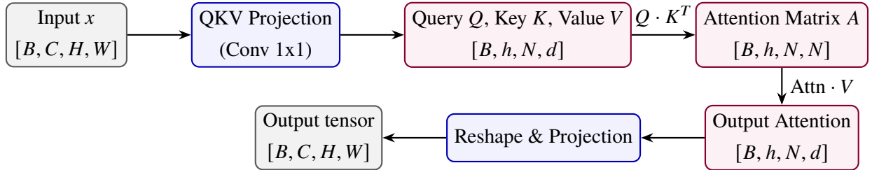
Hình 4.8: Chi tiết luồng xử lý và sự biến đổi kích thước tensor trong module Attention.
