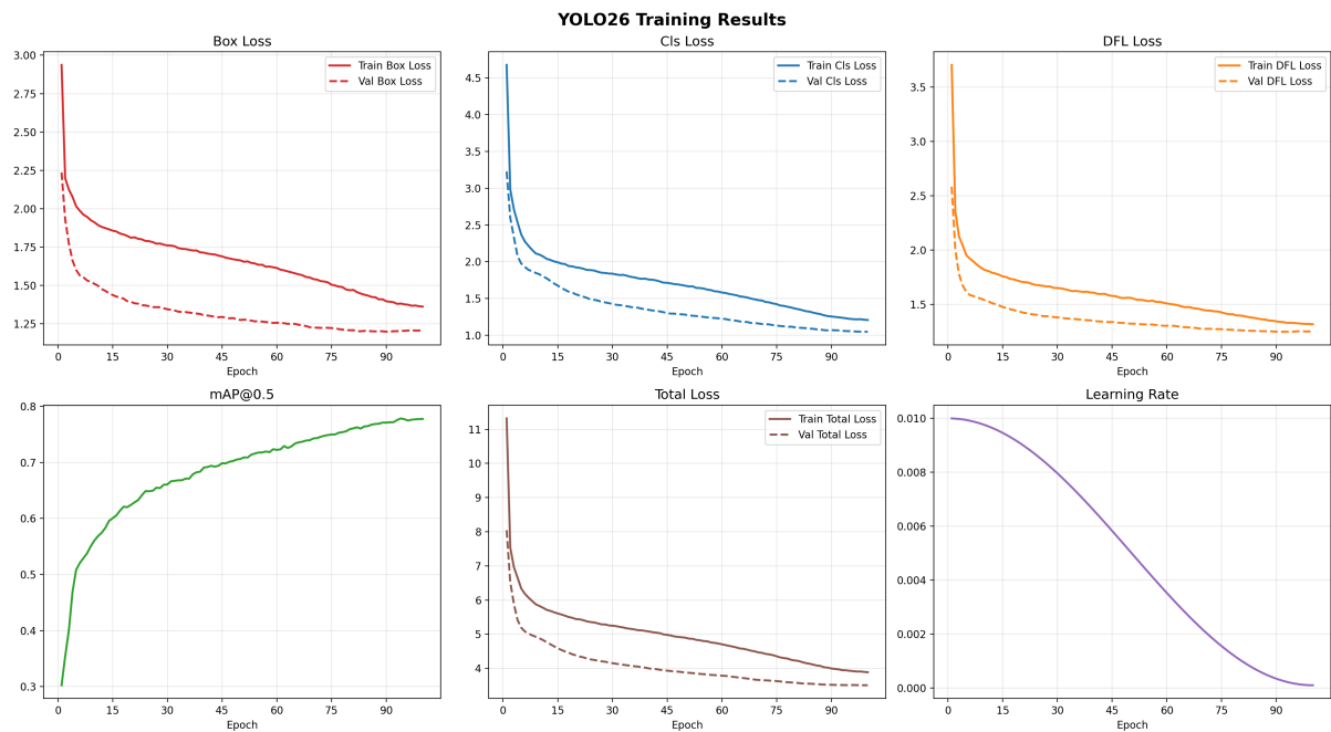
Hình 7.1: Biểu đồ các đường loss và chỉ số đánh giá (metrics) trong quá trình huấn luyện YOLO26 Custom last run qua 100 epochs.
