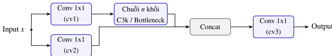
Hình 4.3: Sơ đồ khối C3k — C3 với kernel 3x3 sâu hơn.
