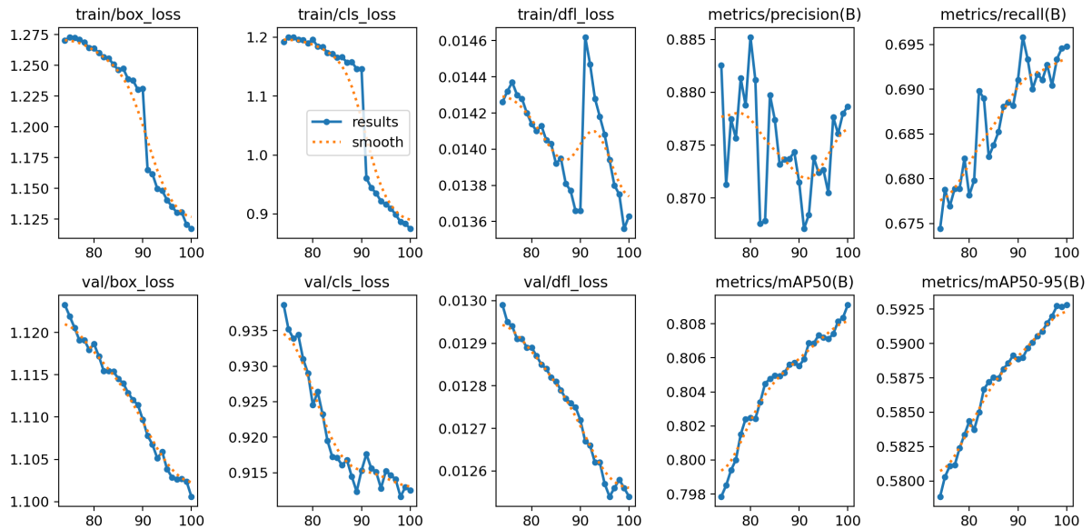
Hình 5.1: Biểu đồ các đường loss và chỉ số đánh giá (metrics) trong quá trình huấn luyện YOLO26 gốc qua 100 epochs.
