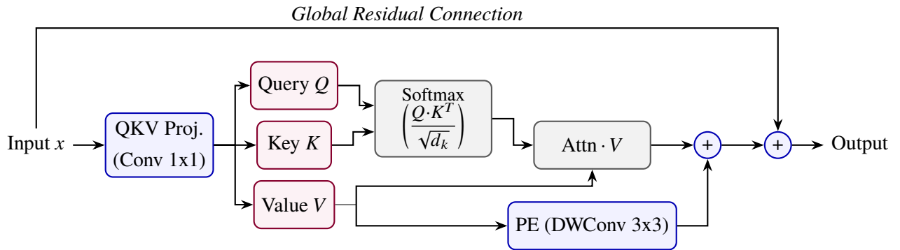
Hình 4.7: Sơ đồ khối Attention với QKV projection và Position Encoding.
