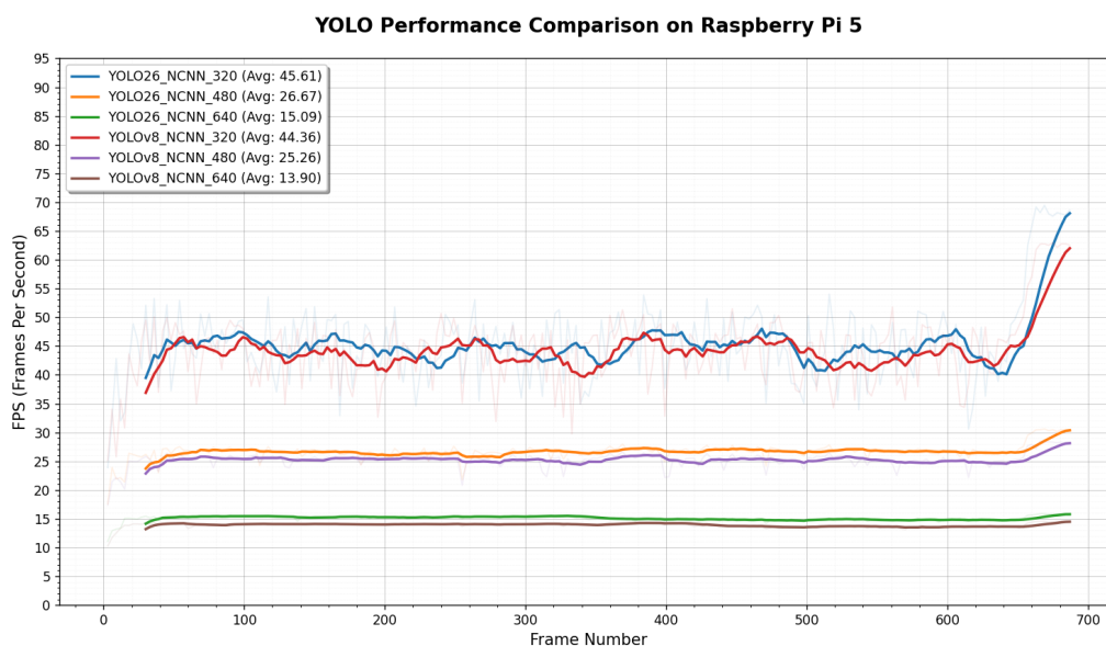
Hình 7.3: Biểu đồ so sánh tốc độ xử lý (FPS) giữa YOLO26 NCNN và YOLOv8 NCNN trên Raspberry Pi 5 ở các độ phân giải 320, 480 và 640.
