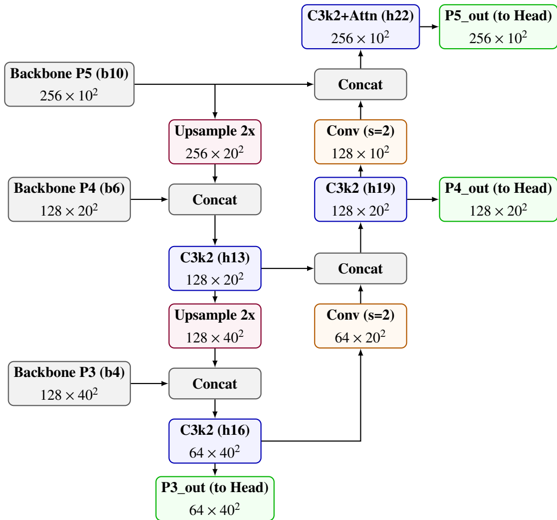
Hình 4.14: Kiến trúc tổng hợp đặc trưng Neck (FPN + PAN) của YOLO26n với kích thước đặc trưng chi tiết cho ảnh đầu vào 320 \times 320 .
