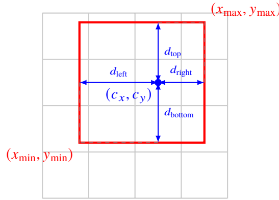
Hình 4.16: Cơ chế giải mã tọa độ bounding box theo khoảng cách LTRB từ tâm ô lưới (c_x, c_y) .
