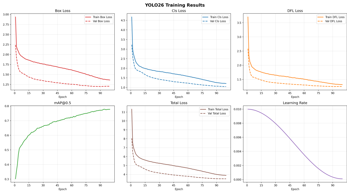
Hình 7.1: Biểu đồ các đường loss và chỉ số đánh giá (metrics) trong quá trình huấn luyện YOLO26 gốc qua 100 epochs.
