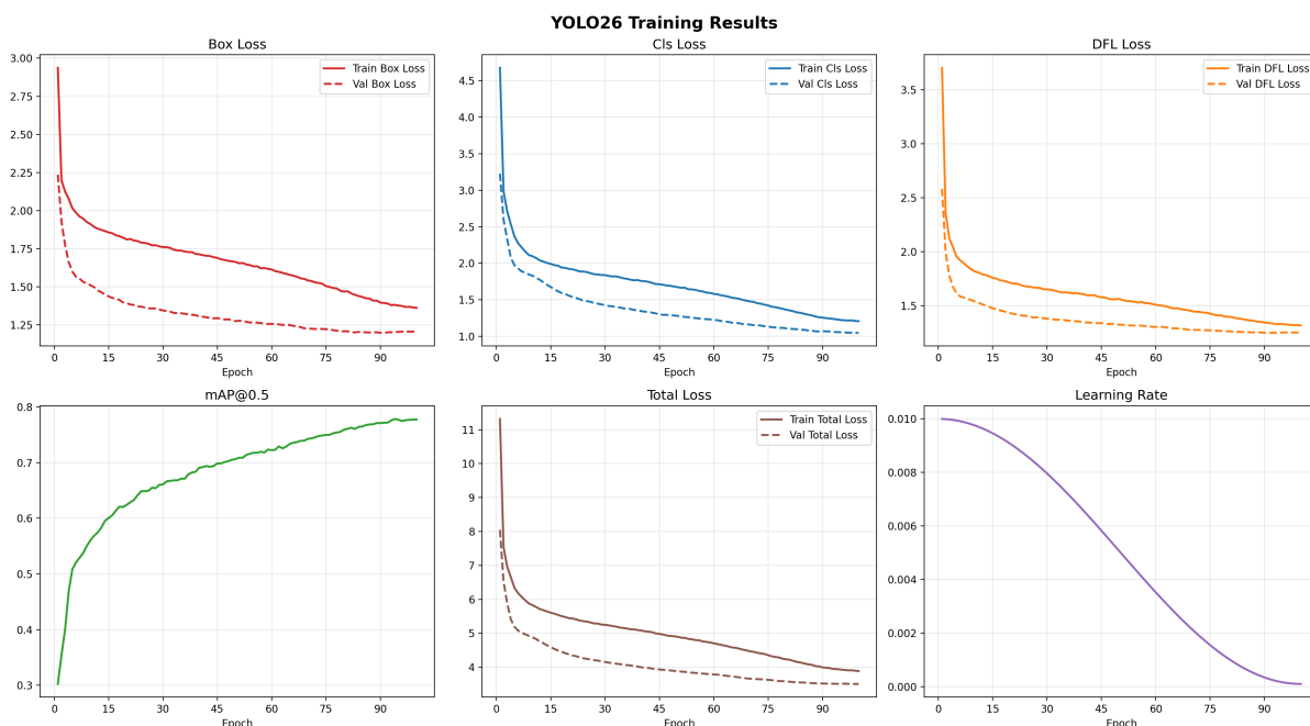
Hình 5.1: Biểu đồ các đường loss và chỉ số đánh giá (metrics) trong quá trình huấn luyện YOLO26 gốc qua 100 epochs.
