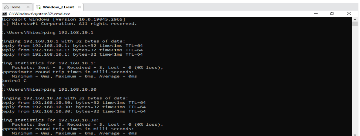
Hình 5.2. Windows Client kiểm tra kết nối đến pfSense và Kali Linux
