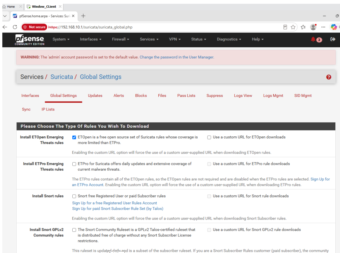
Hình 5.10. Cấu hình bộ luật và cơ chế cập nhật của Suricata IDS
