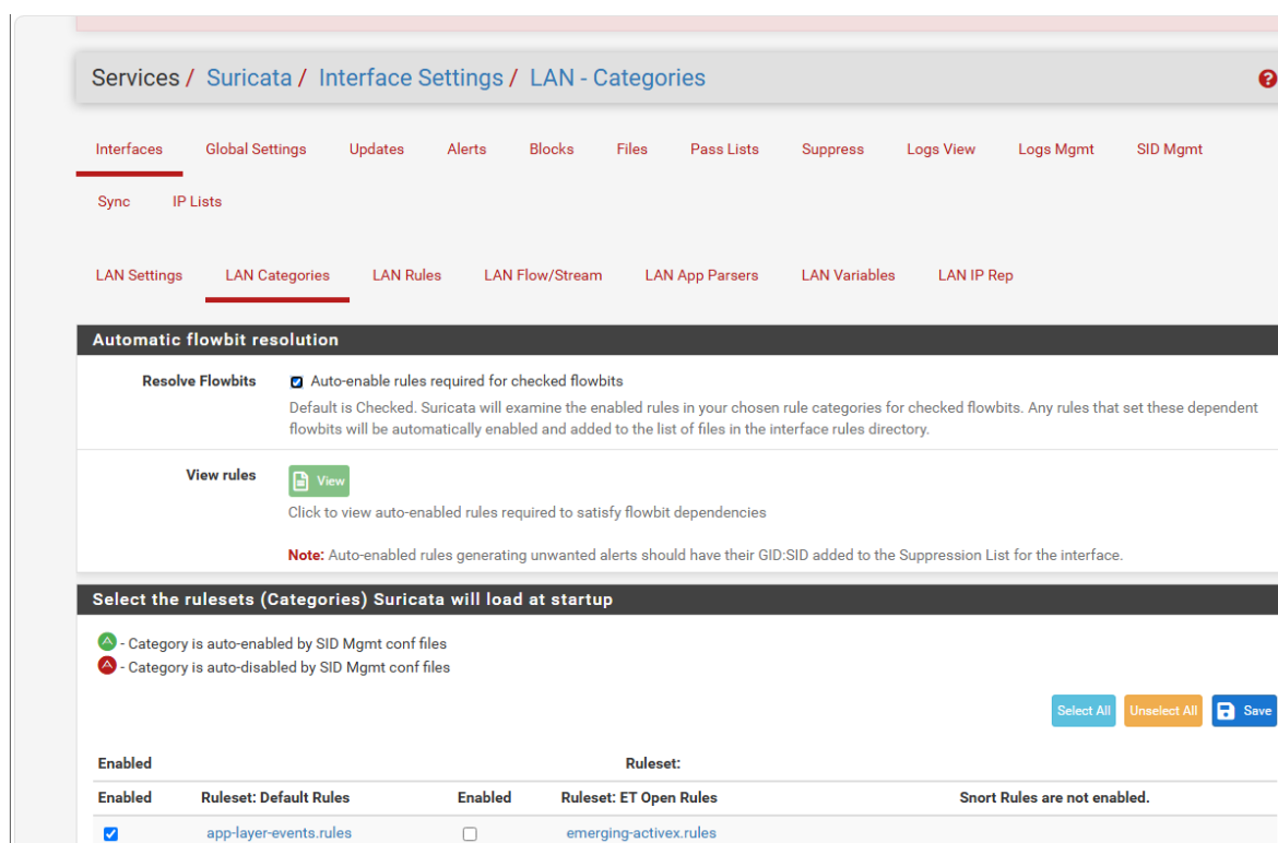
Hình 5.15. Giao diện lựa chọn nhóm luật phát hiện xâm nhập cho Suricata
