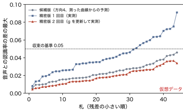
図 8 [未来日記 F6-3・planned] 候補版, 精密版 1 回目, 精密版 2 回目の, 札ごとの残差 (音声との認識率の差の最大). 残差の小さい順に並べた. 破線は収束の基準 0.05 である.
