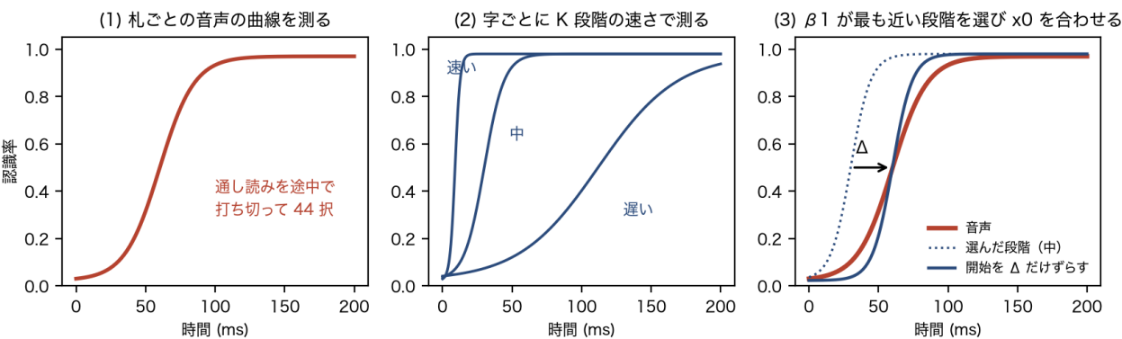
図 4 方向 4 (候補版) の仕組みの模式図. (1) 札ごとの音声の曲線と, (2) 速さを K 段階に変えて測定した文字の曲線を用意し, (3) 傾き \beta_1 が最も近い段階を選択して開始を \Delta だけずらすと, 音声の曲線に重なる. 見せるアニメーションは (2) で測定したものそのものである.
