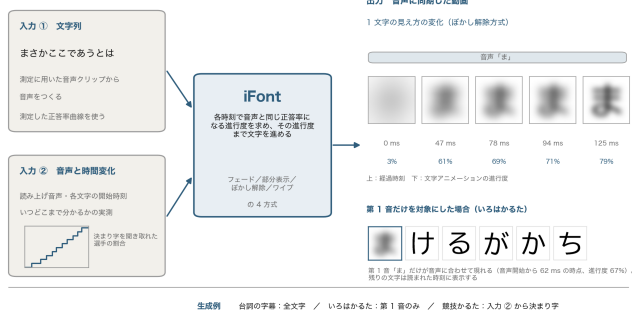
図 1 timeFont の生成の仕組み (先行する報告 [2] より再掲. 図中の iFont は timeFont の旧称). 文字列と, 音声および各字の曲線を入力し, 各時刻で音声と同じ認識率になる進捗度まで文字を進める. 下段は 1 音目だけを対象にした場合である.
