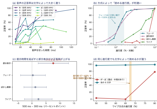
図 2 かな 1 文字の測定の結果 (先行する報告 [2] より再掲). (a) 音声の正答率は字によって大きく異なる. (b) 方式によって読める進行度が異なる. (c) 提示時間を延ばすと部分表示だけ正答率が上がる. (d) ワイプでは濁点の出現位置で正答率が跳ね上がる.
