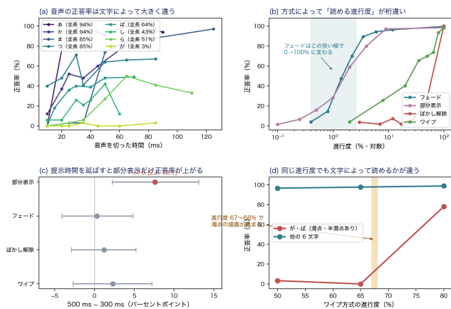
図 2 かな 1 文字の測定の結果 (先行する報告 [2] より再掲). (a) 音声の正答率は字によって大きく異なる. (b) 方式によって読める進行度が異なる. (c) 提示時間を延ばすと部分表示だけ正答率が上がる. (d) ワイプでは濁点の出現位置で正答率が急に上昇する.
