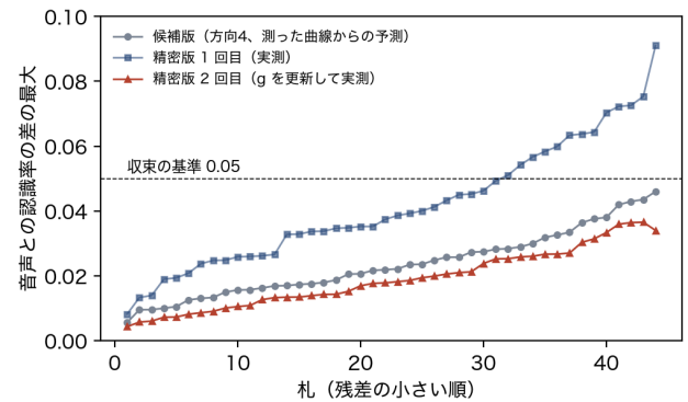
図 8 候補版, 精密版 1 回目, 精密版 2 回目の、札ごとの残差 (音声との認識率の差の最大). 残差の小さい順に並べた. 破線は収束の基準 0.05 である.
