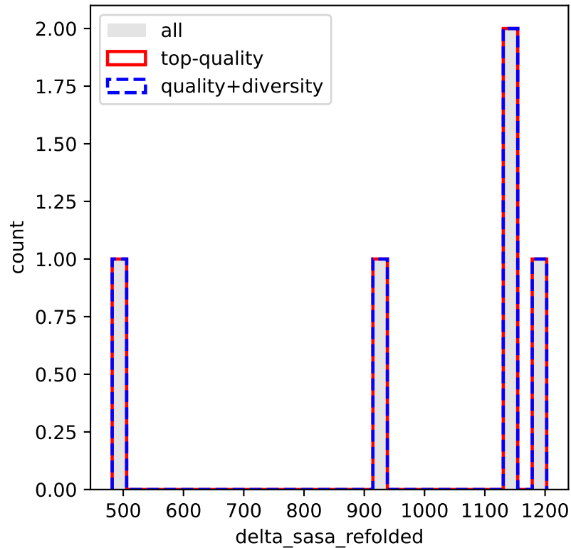
delta_sasa_refolded
