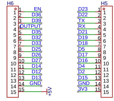
排针引出
