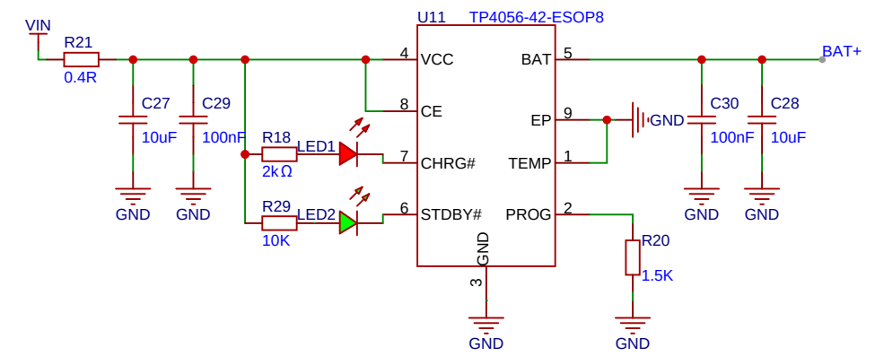
TP4056充电电路
