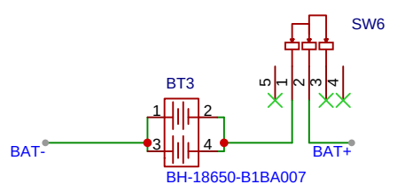
18650 电池
