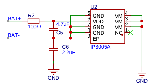
IP3005A 锂电池保护电路
