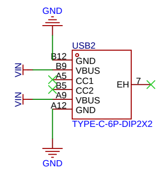
TYPEC电池充电
