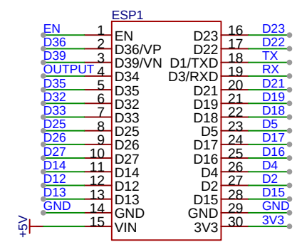
ESP-32主控
