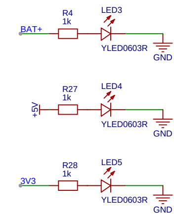
电源指示灯
