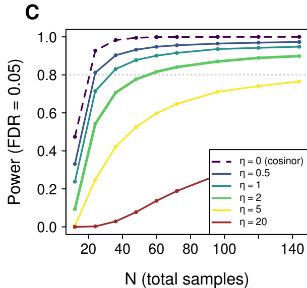
\omega_g \sim B(1, \eta)
