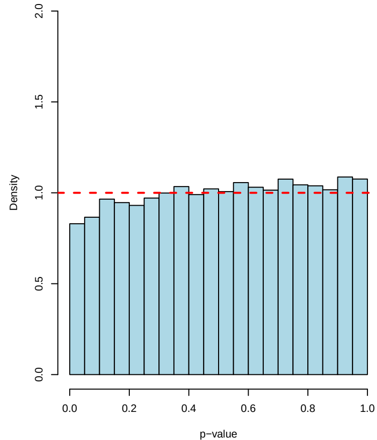
DA p-values under null (n=60)
