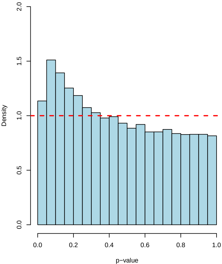
DR p-values under null (n=60)
