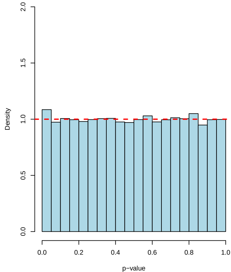
DP p-values under null (n=60)
