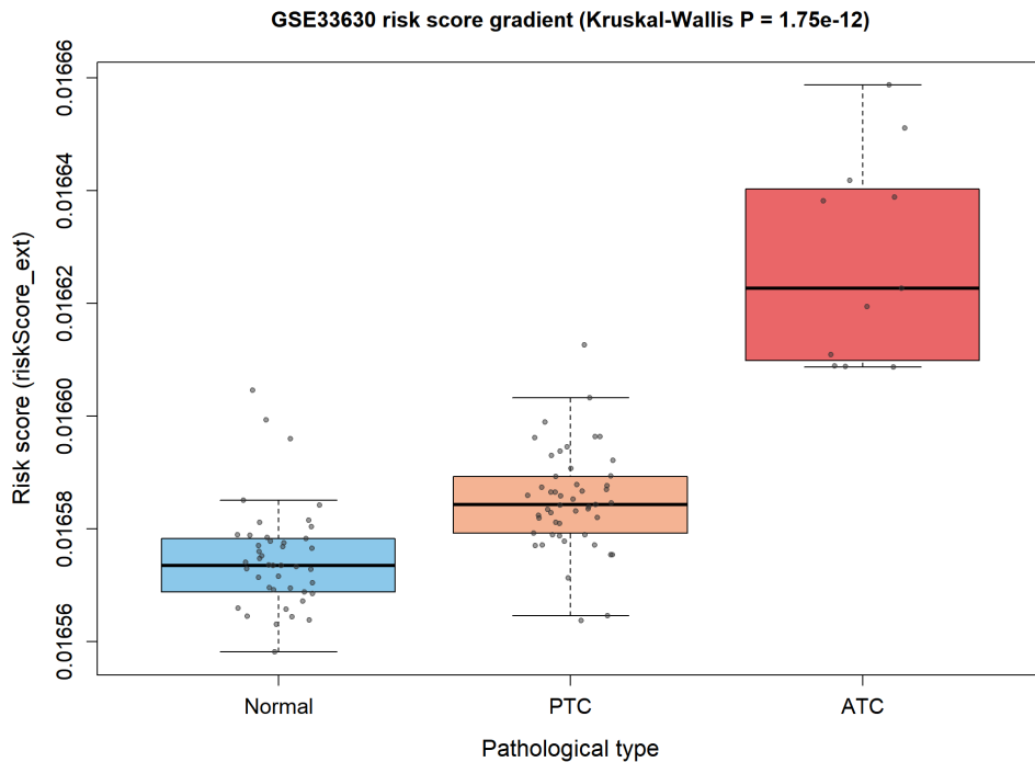
图 7 GSE33630 中风险评分病理类型梯度 (Kruskal-Wallis P = 1.75 \times 10^{-12} )
