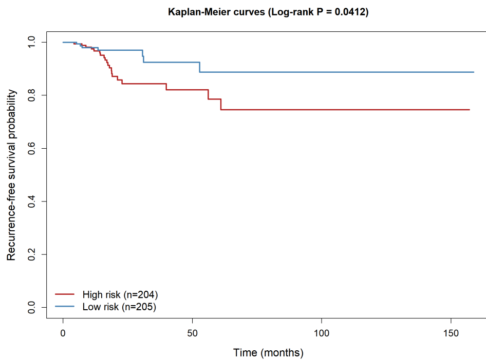
图 3 高、低风险组无复发生存 Kaplan-Meier 曲线 (Log-rank P = 0.0412)
