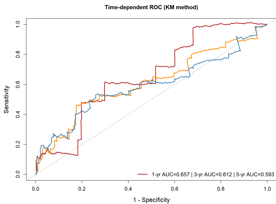
图 4 时间依赖 ROC 曲线 (1/3/5 年 AUC = 0.657/0.612/0.593, KM 法)
