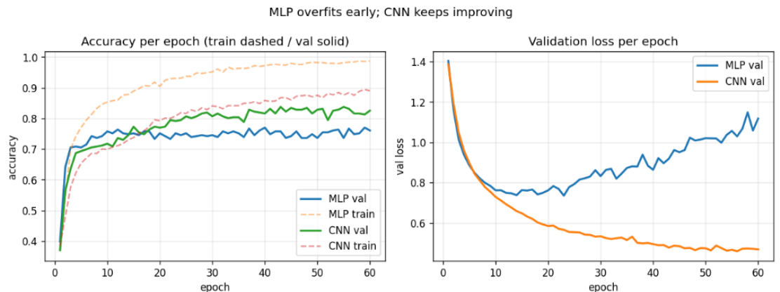
Figure 3: 에폭별 학습 곡선 (MLP vs CNN) - MLP는 20에폭 이후 val loss 재상승(과적합), CNN은 60에폭까지 꾸준히 개선
