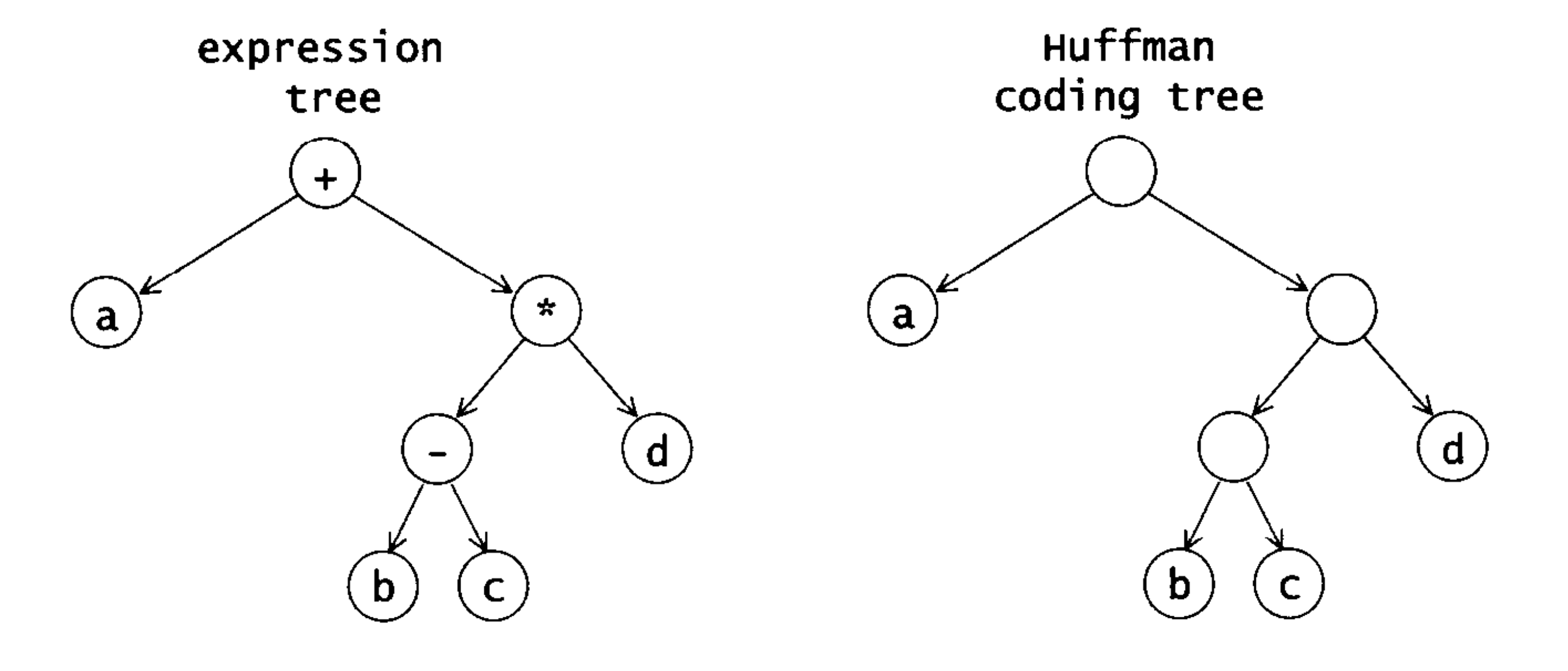
图 5-3 二叉树的应用
