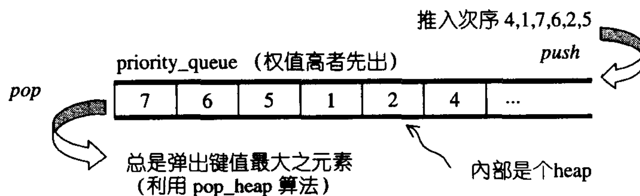
图 4-24 priority_queue
