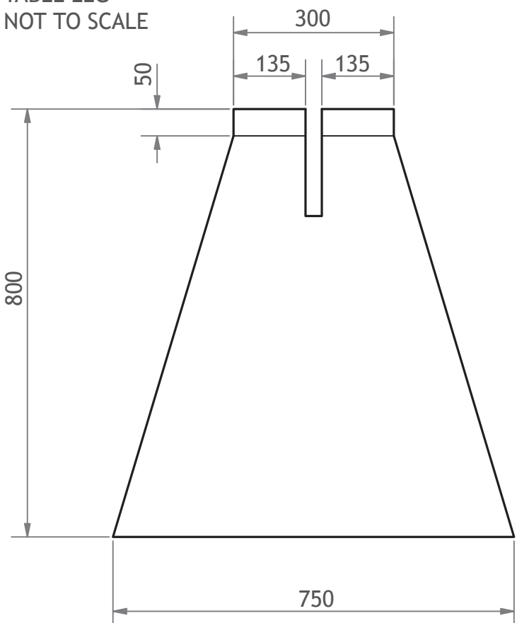
ELEVATION
