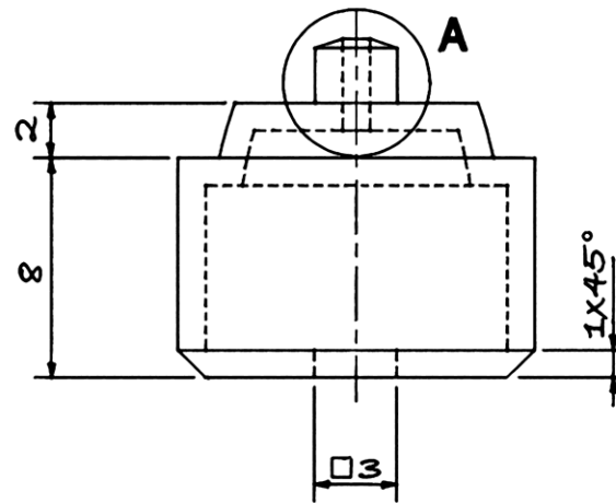
End Elevation
