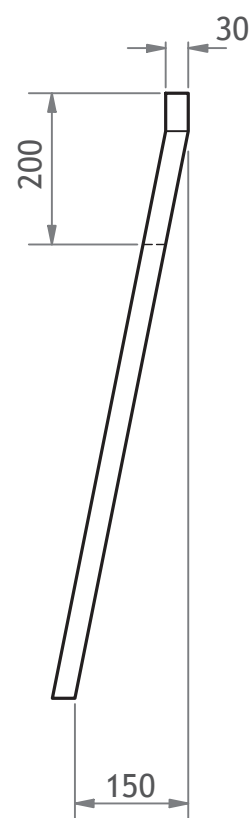
END ELEVATION
