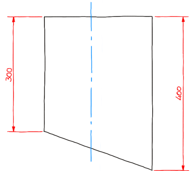
END ELEVATION
