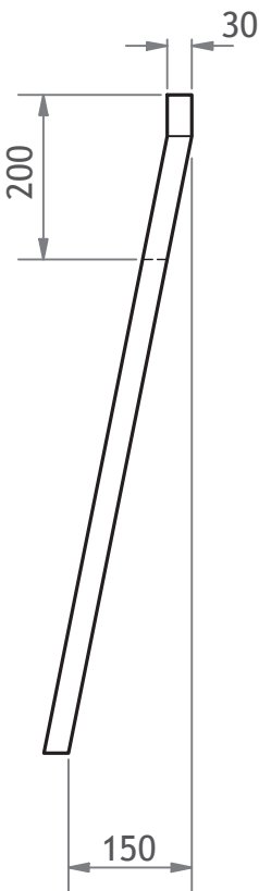
END ELEVATION
