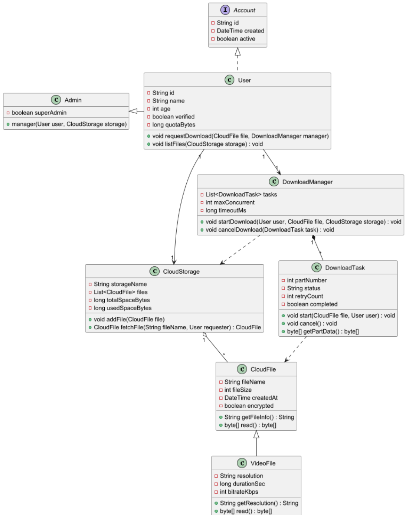
Рисунок 1 - Диаграмма классов
