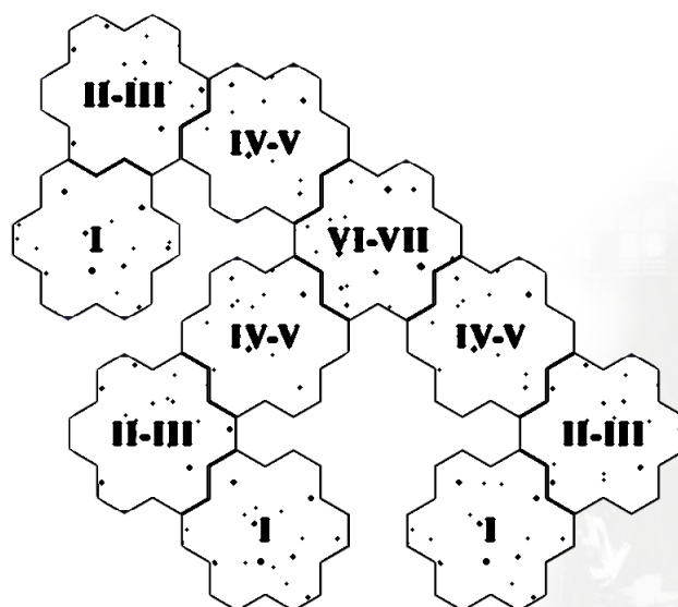
3-PLAYER SCENARIO
