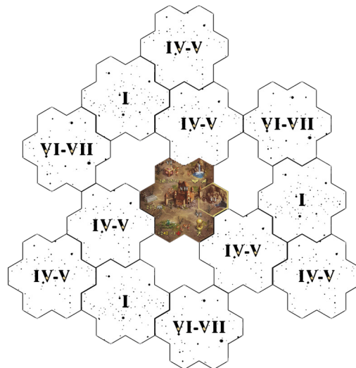
3-PLAYER SCENARIO
