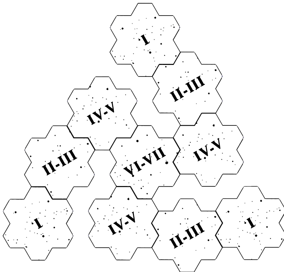
3-PLAYER SCENARIO
