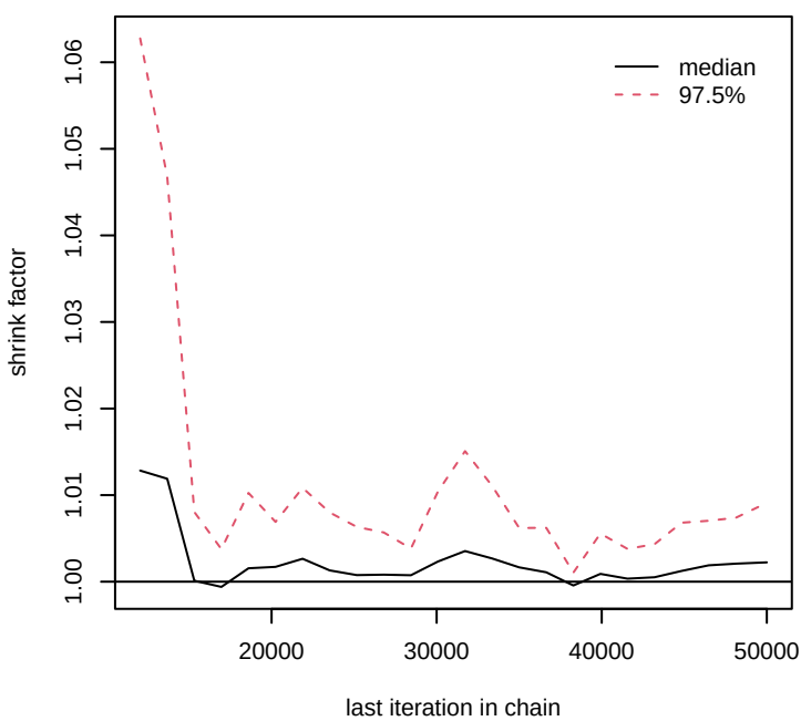
test.spec[1]
