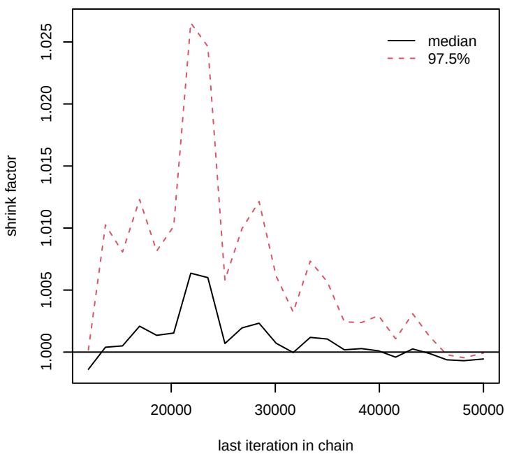
rho
