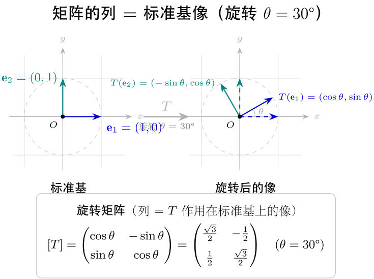
图 17: 标准基的像就是矩阵 T 的列（旋转 30^\circ 示例）
