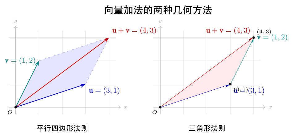
图 1: 平行四边形法则与三角形法则示意
