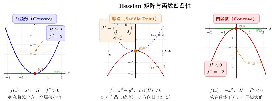
图 23-2: Hessian 与凹凸
