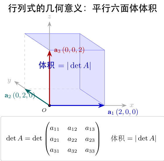
图 10: 三列向量张成的平行六面体体积 = |\det A|
