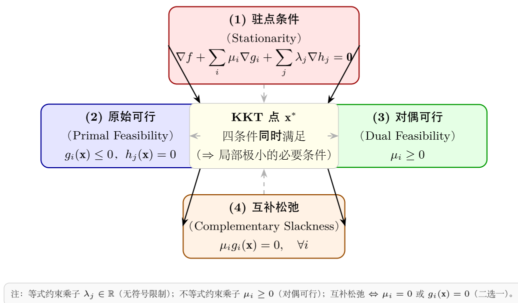
图 13: 原始可行 + 对偶可行 + 互补松弛 + 驻点
