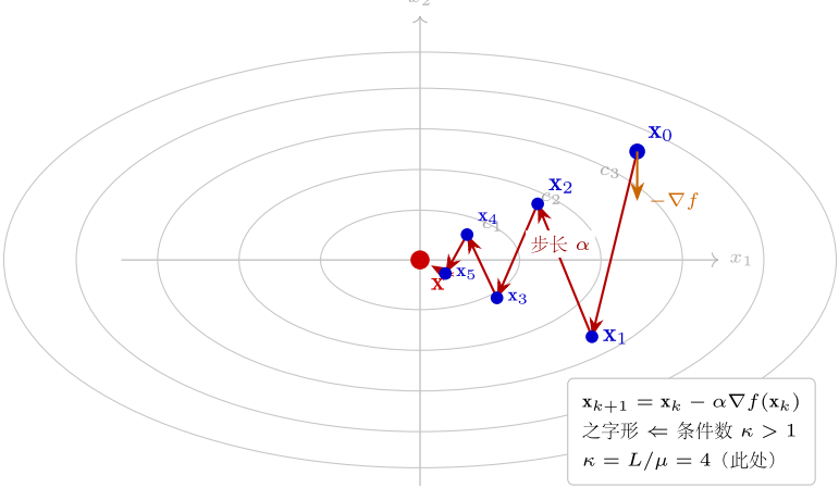
梯度下降轨迹：椭圆等高线 + 之字形收敛
