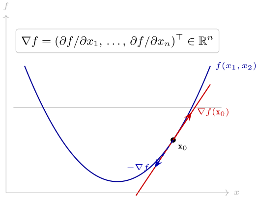
梯度 = 偏导数列向量
