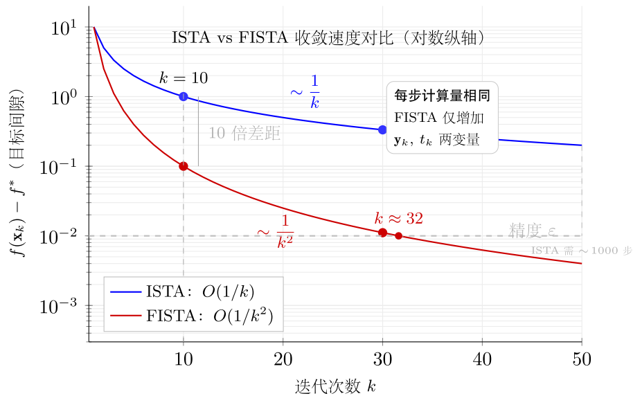
图 21: O(1/k) vs O(1/k^2) 对比
