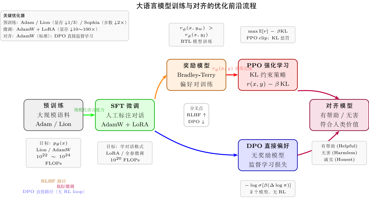
图 39: 预训练 → SFT → RLHF/DPO → 对齐
