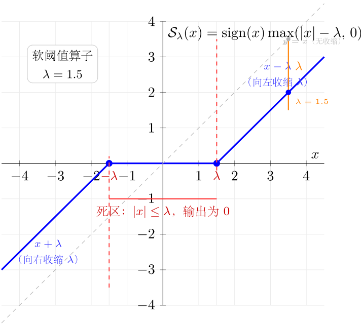
图 20: \text{prox}_{\lambda \|\cdot\|_1} 三段折线
