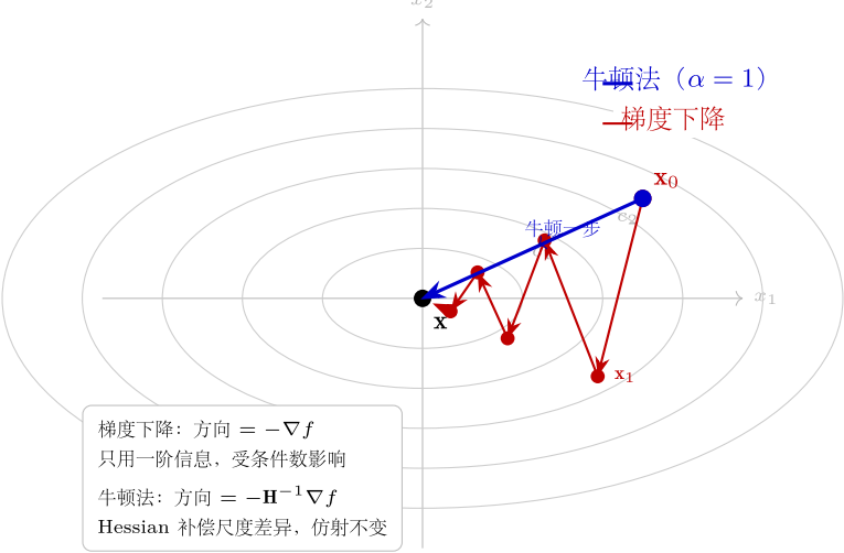
图 9: 相同椭圆等高线，GD 之字形多步收敛 vs 牛顿法一步直达
