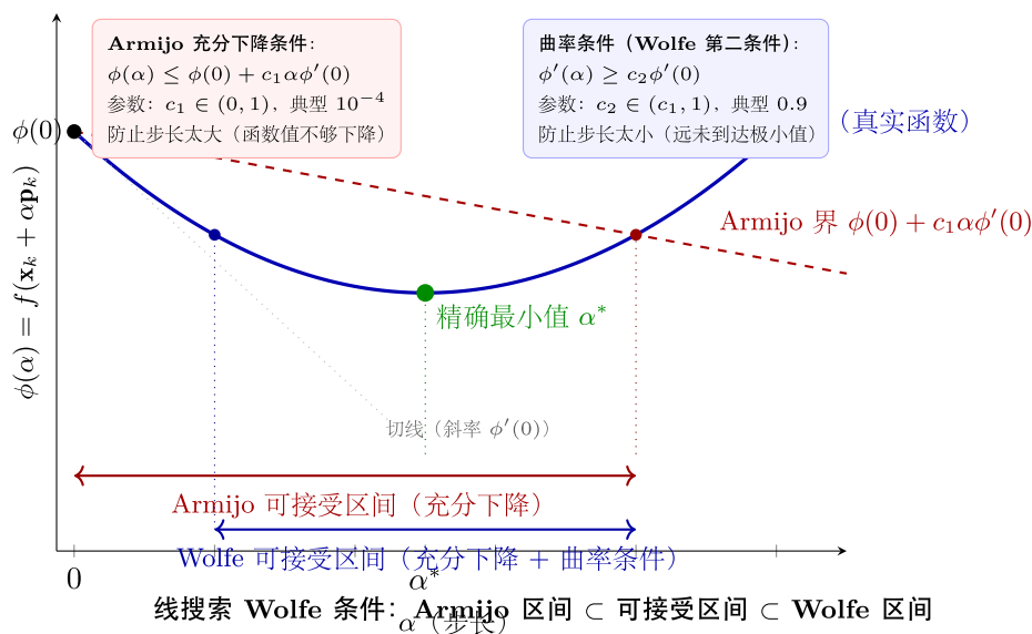
图 22: Armijo 下降 + 曲率改善
