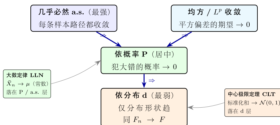
图 19: 随机收敛的四种模式与强弱层次：a.s. 与 L^p 均蕴含依概率，依概率蕴含依分布
