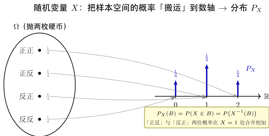
图 17: 随机变量把样本空间上的概率搬运到数轴，得到分布
