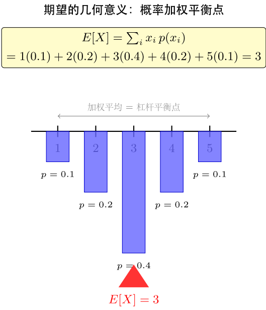
图 9: 期望的几何意义：加权平均等于杠杆平衡点
