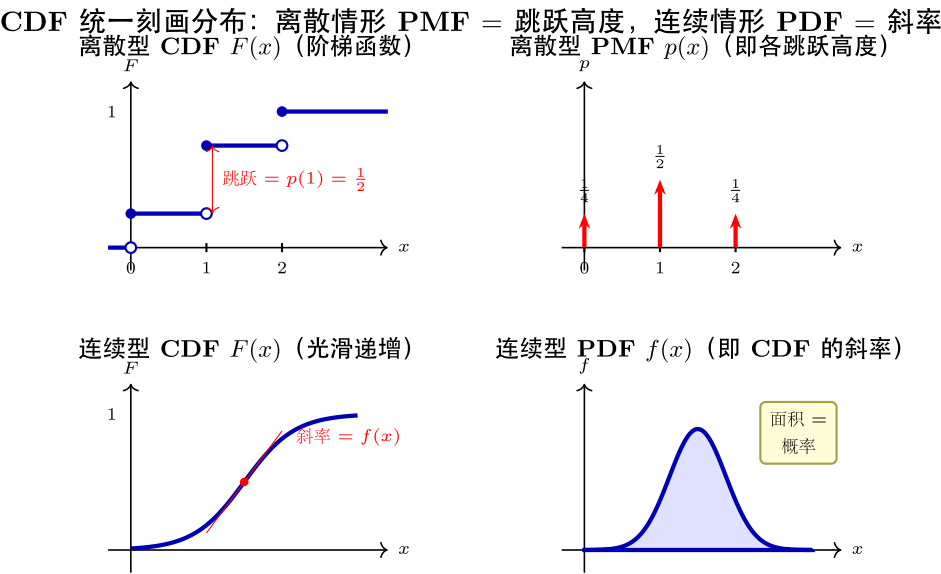
图 18: CDF 统一刻画分布：离散情形 PMF 是 CDF 的跳跃高度，连续情形 PDF 是 CDF 的斜率
