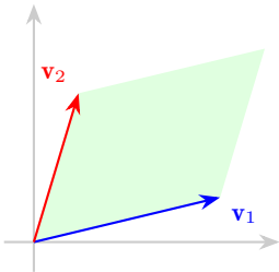
线性无关 张成整个平面
