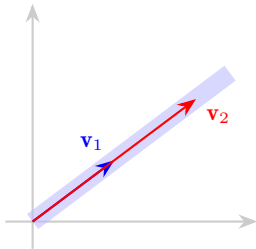
线性相关 只张成一条线
