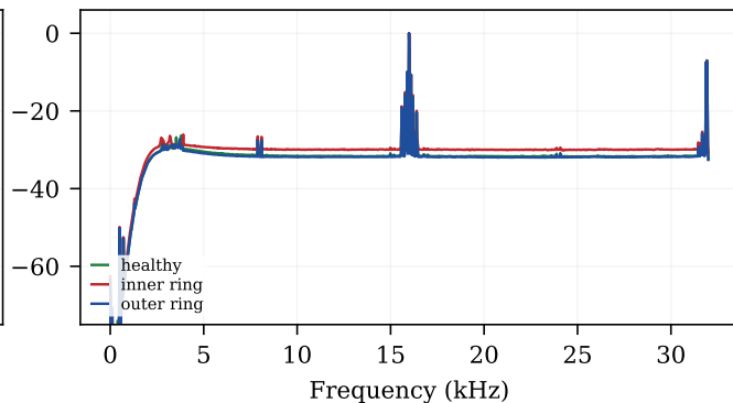
(d) Paderborn, 2 kHz high-pass (rig-tone control)
