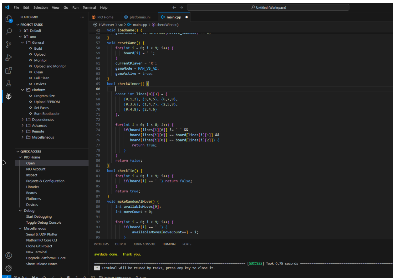
Рис. 2. Середовище розробки у VS code з розширенням PlatformIo
