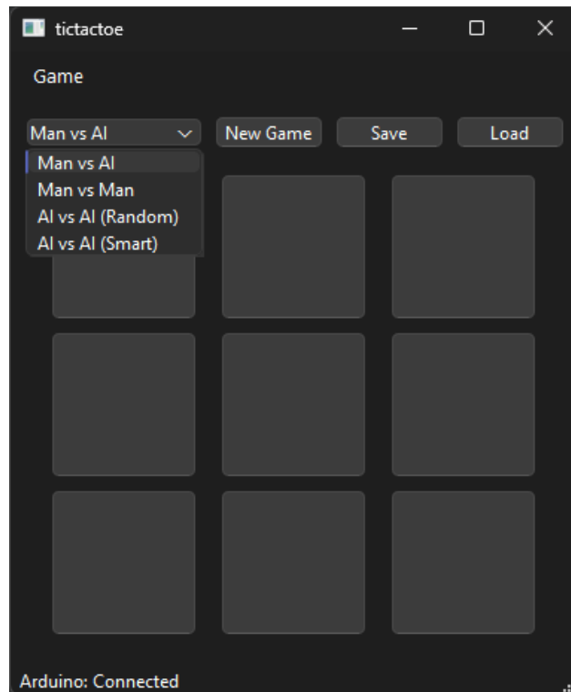
Рис. 3. Графічний дизайн гри ТікТакТое
