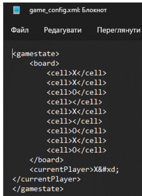
Рис. 6. Файл game_config.xml
