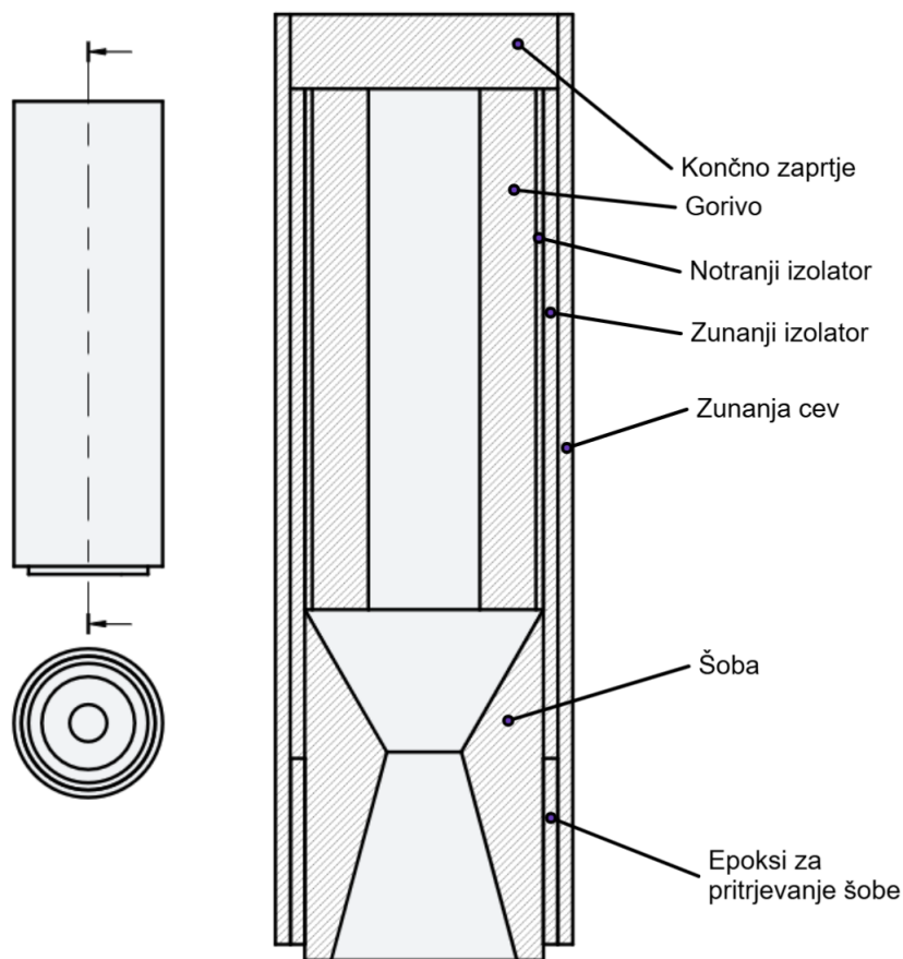
Slika 6: Shema motorja
