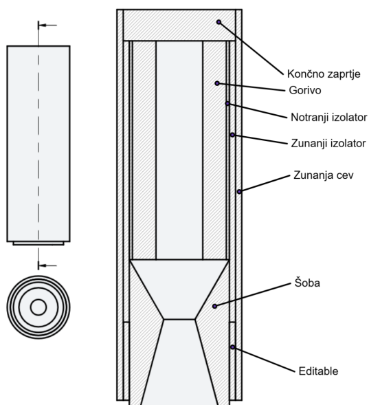
Slika 5: Shema motorja
