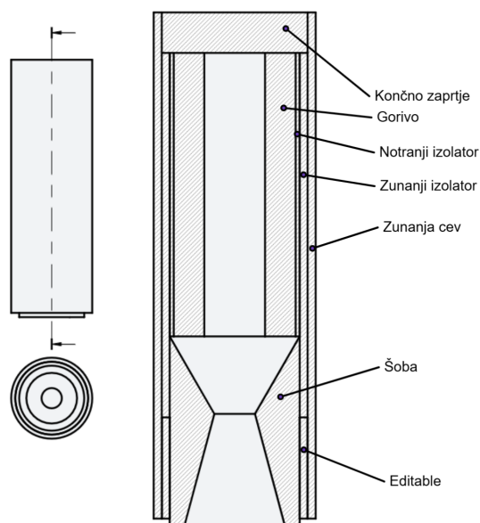
Slika 5: Shema motorja
