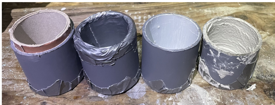
Slika 2: Prvi test: karton, tekstilni lepilni trak, kontrola, cement
