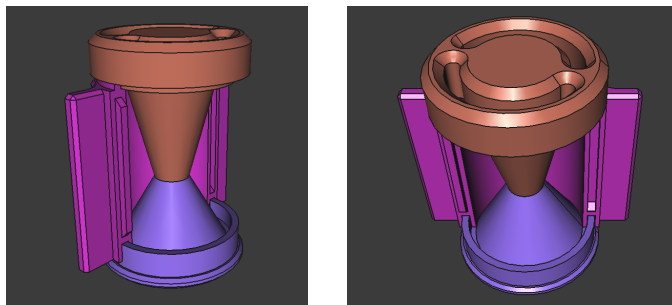
Slika 6: Načrt modelčka za ulivanje šob
